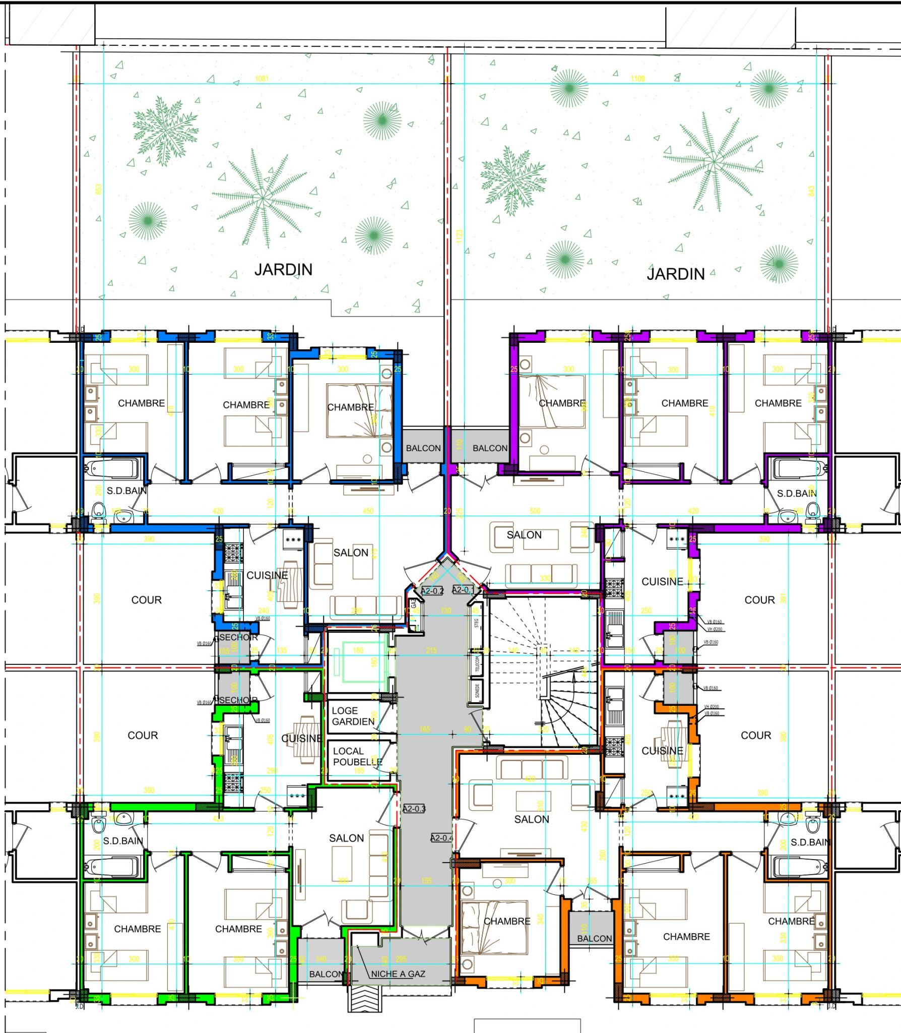
BLOC A.2 PLAN REZ-DE-CHAUSSEE
