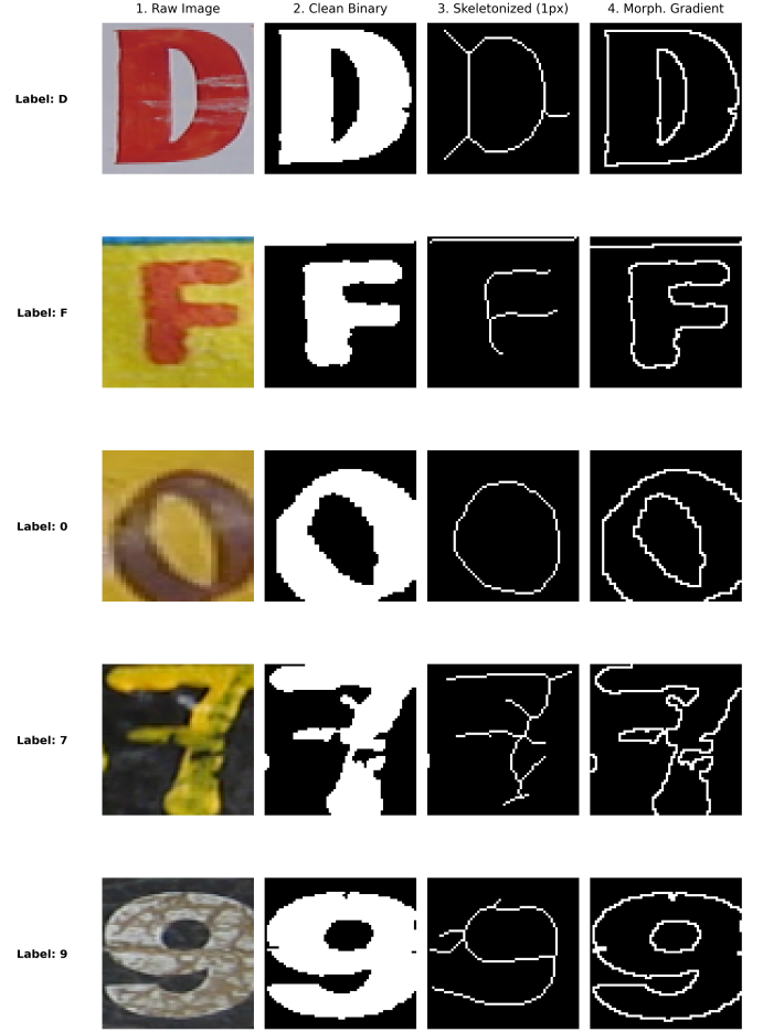
Fig. 2. Perbandingan tahapan prapemrosesan: (1) Citra Asli, (2) Binerisasi Bersih (Otsu + Hole-filling \leq 35 px), (3) Skeletonisasi 1 piksel (metode konvensional), (4) Morphological Gradient / kontur (metode yang diusulkan).
