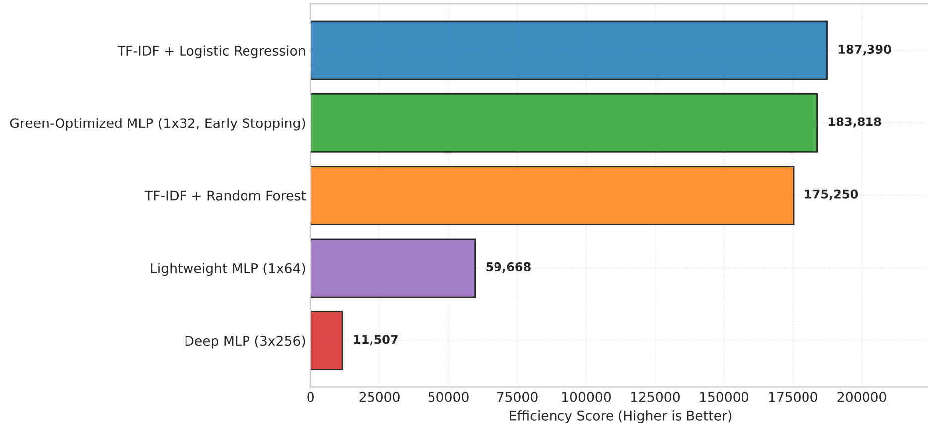
Green AI Efficiency Score (Accuracy % per Gram CO_2eq )
