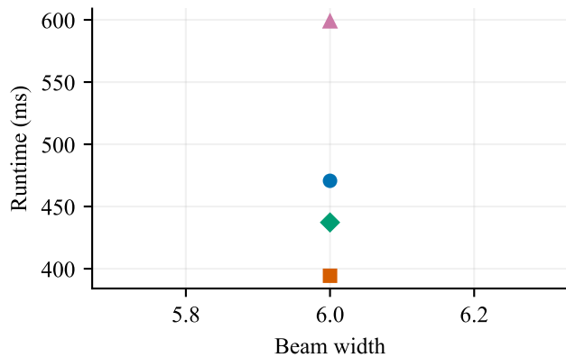
Runtime (ms)
