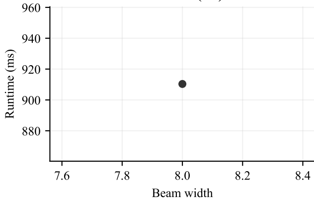
Runtime (ms)
