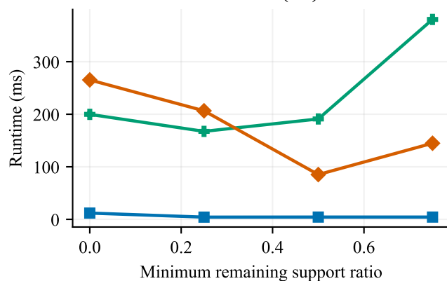
Runtime (ms)
