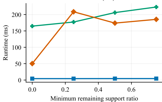
Runtime (ms)
