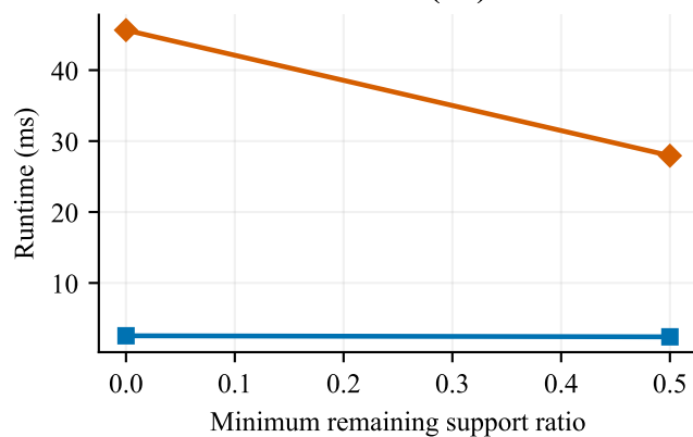
Runtime (ms)
