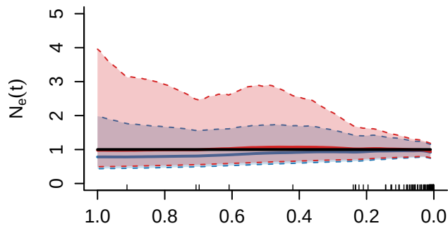
RI-BM
