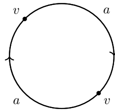
\mathbb{R}P^2
