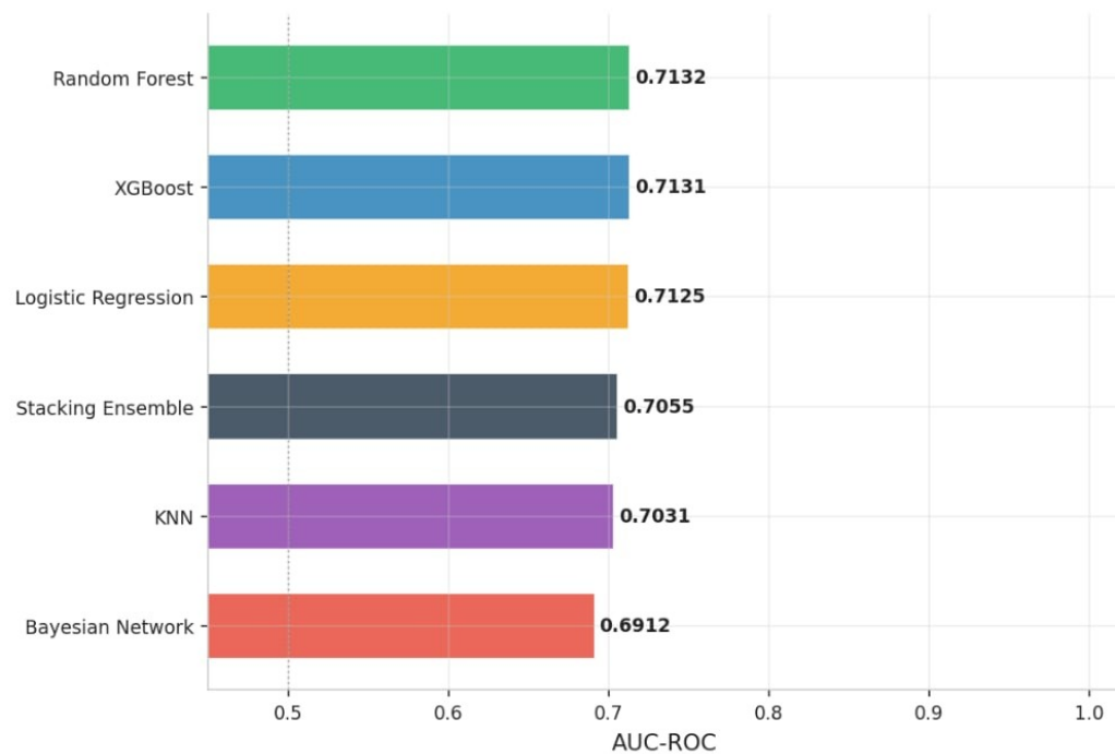
AUC-ROC Comparison
