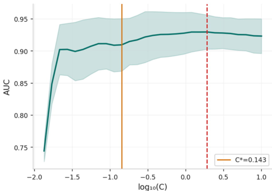
① CV AUC (Max \rightarrow C^* )
