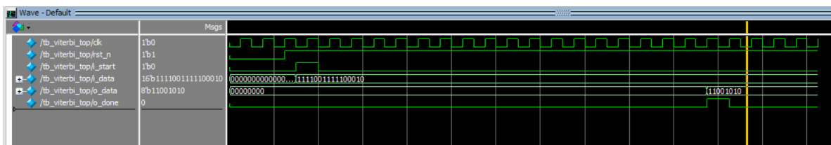
Hình 3.6: Waveform mô phỏng module top
