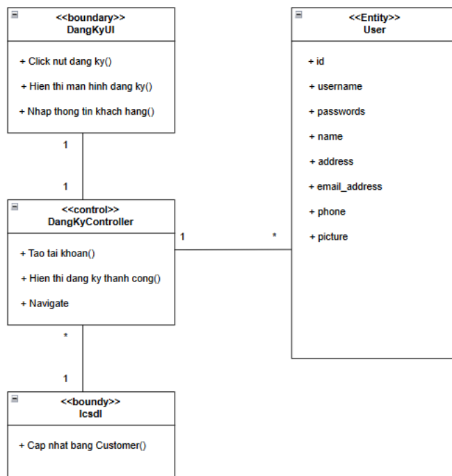
Hình 3-3: Biểu đồ lớp chức năng đăng ký
