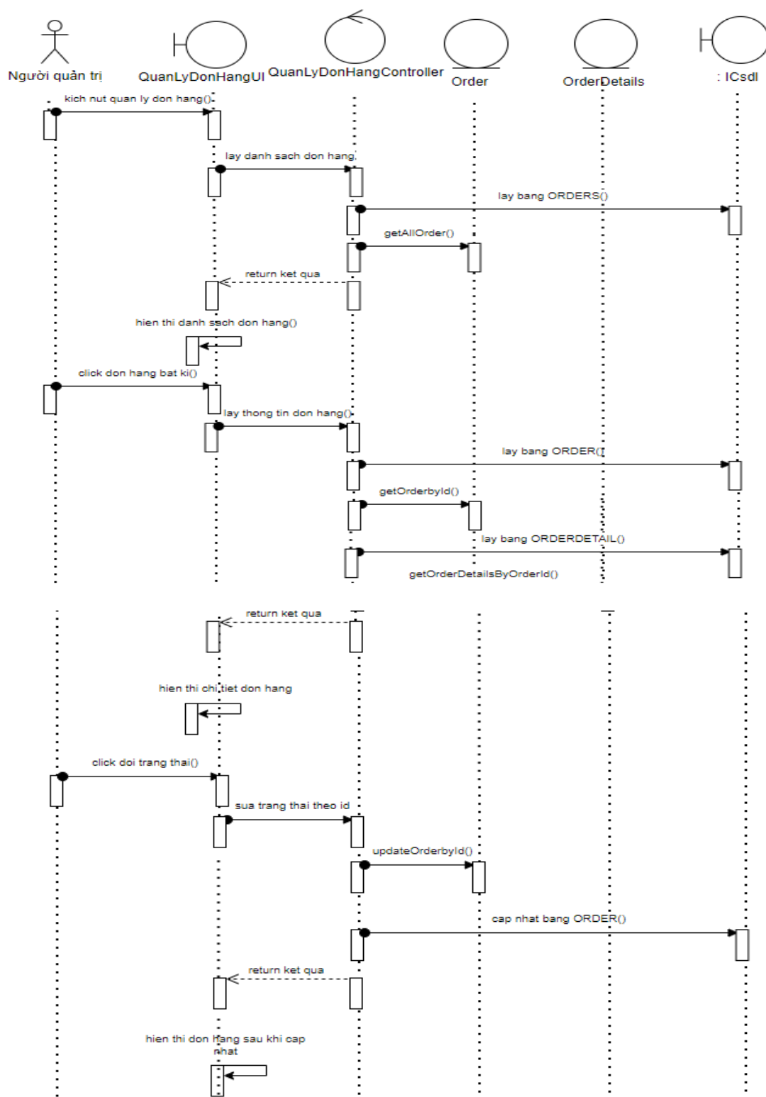
Hình 3-16: Biểu đồ trình tự chức năng đơn hàng
