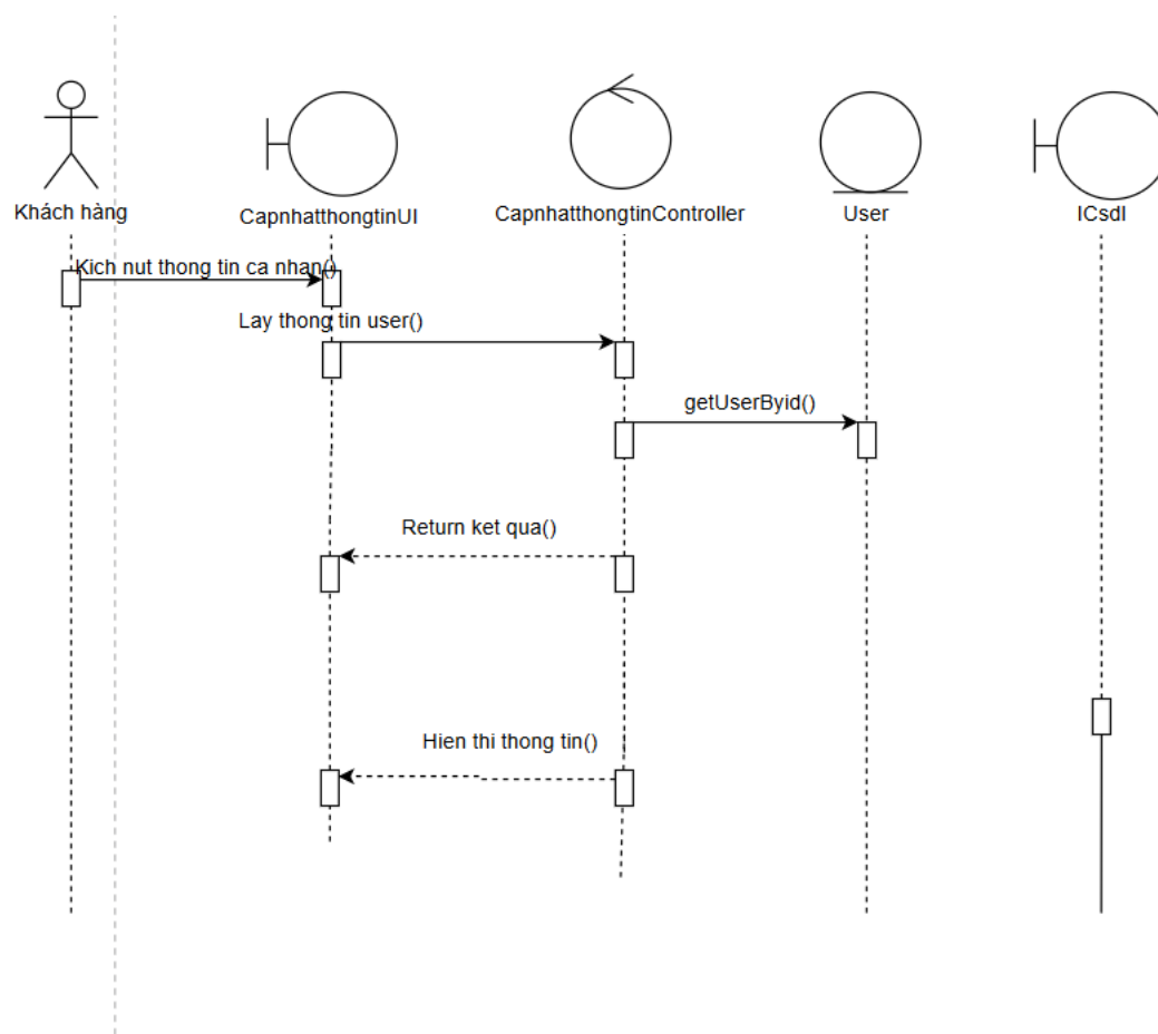
Hình 3-8: Biểu đồ trình tự chức năng cập nhật thông tin
