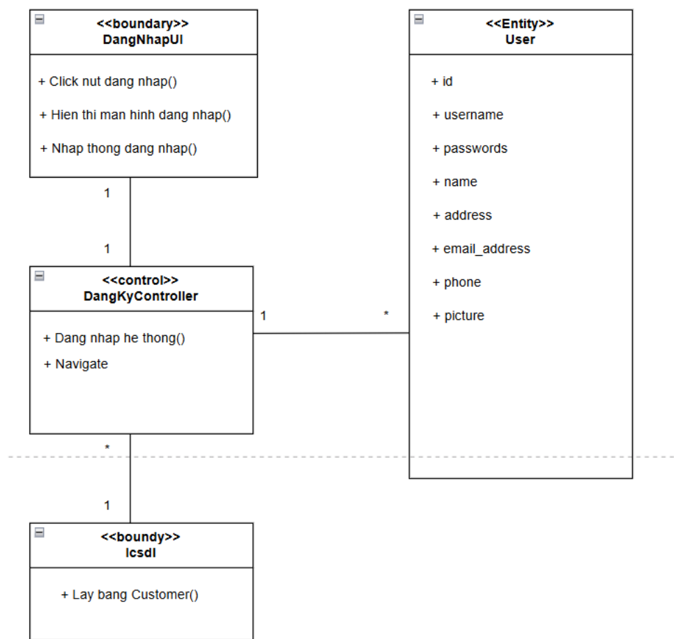
Hình 3-5: Biểu đồ lớp chức năng đăng nhập
