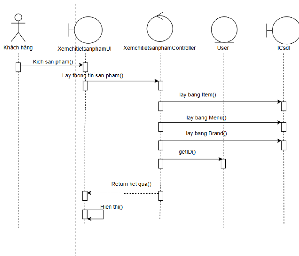
Hình 3-9: Biểu đồ trình tự chức năng xem chi tiết sản phẩm
