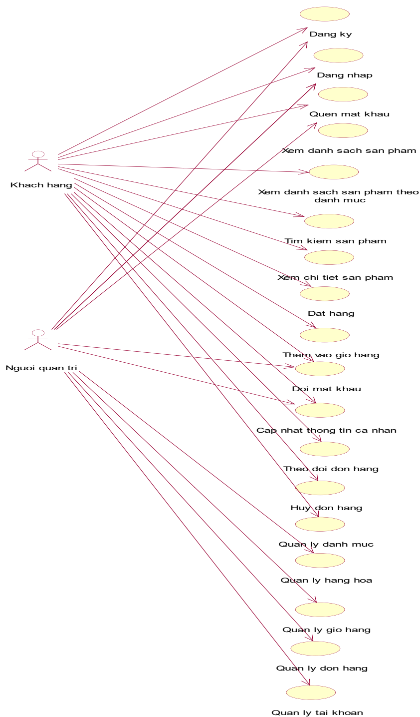
Hình 3-1: Mô hình use case của các tác nhân
