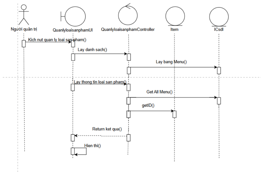
Hình 3-15: Biểu đồ trình tự chức năng quản lý danh mục
