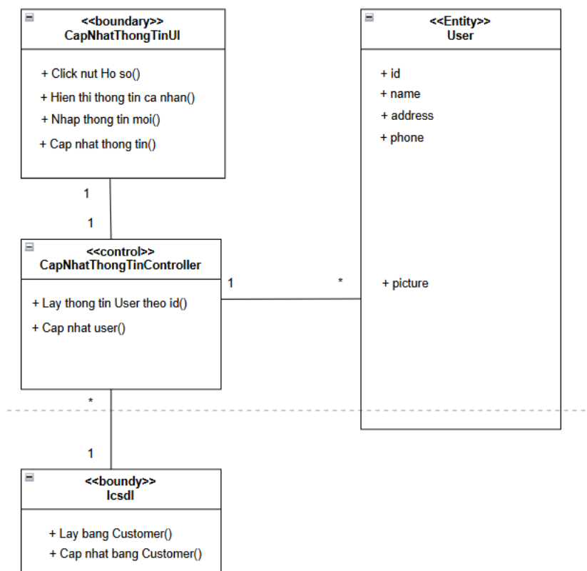
Hình 3-7: Biểu đồ lớp chức năng cập nhật thông tin
