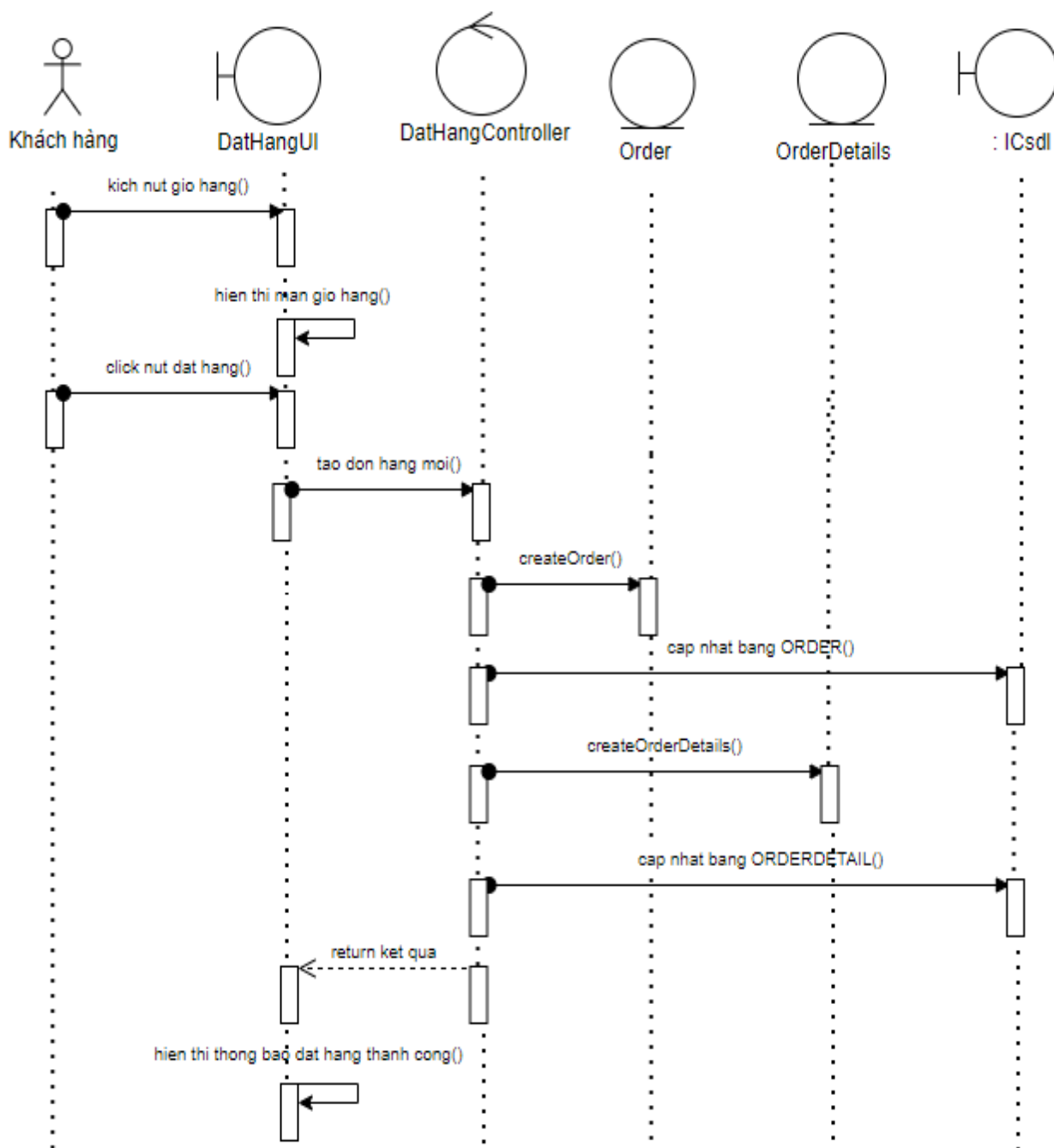
Hình 3-12 :Biểu đồ trình tự chức năng đặt hàng
