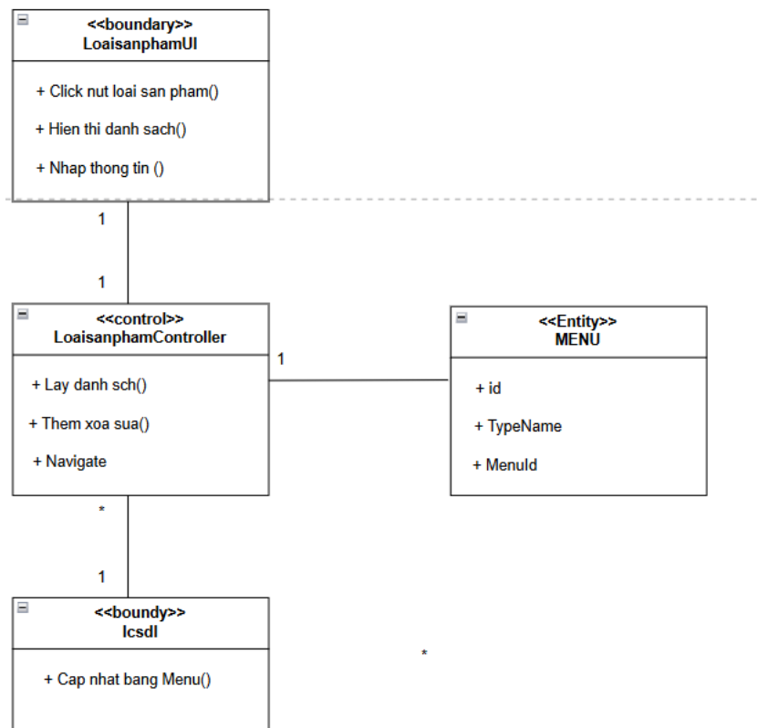
Hình 3-14: Biểu đồ lớp chức năng quản lý loại sản phẩm
