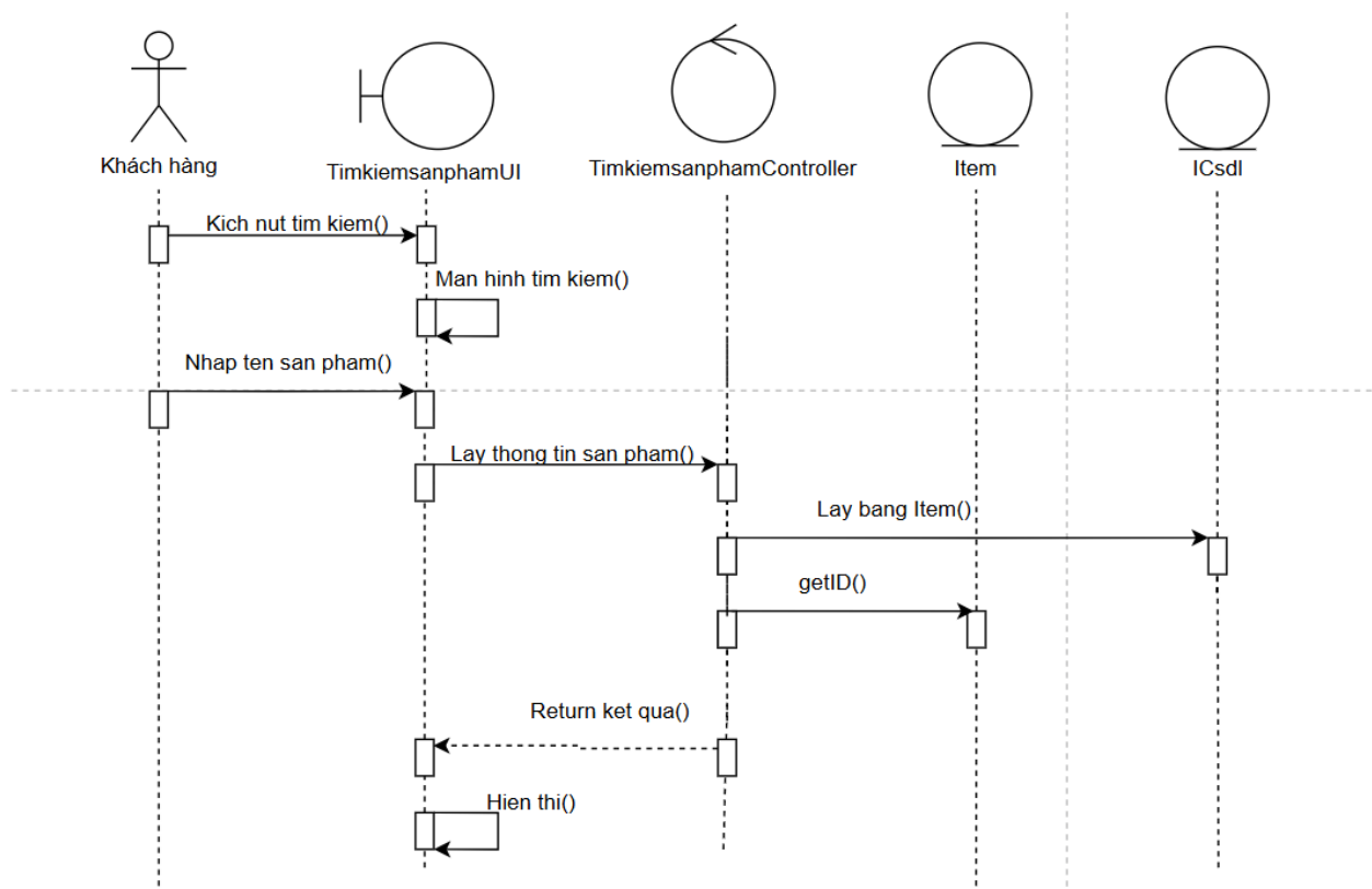
Hình 3-10: Biểu đồ trình tự chức năng tìm kiếm sản phẩm
