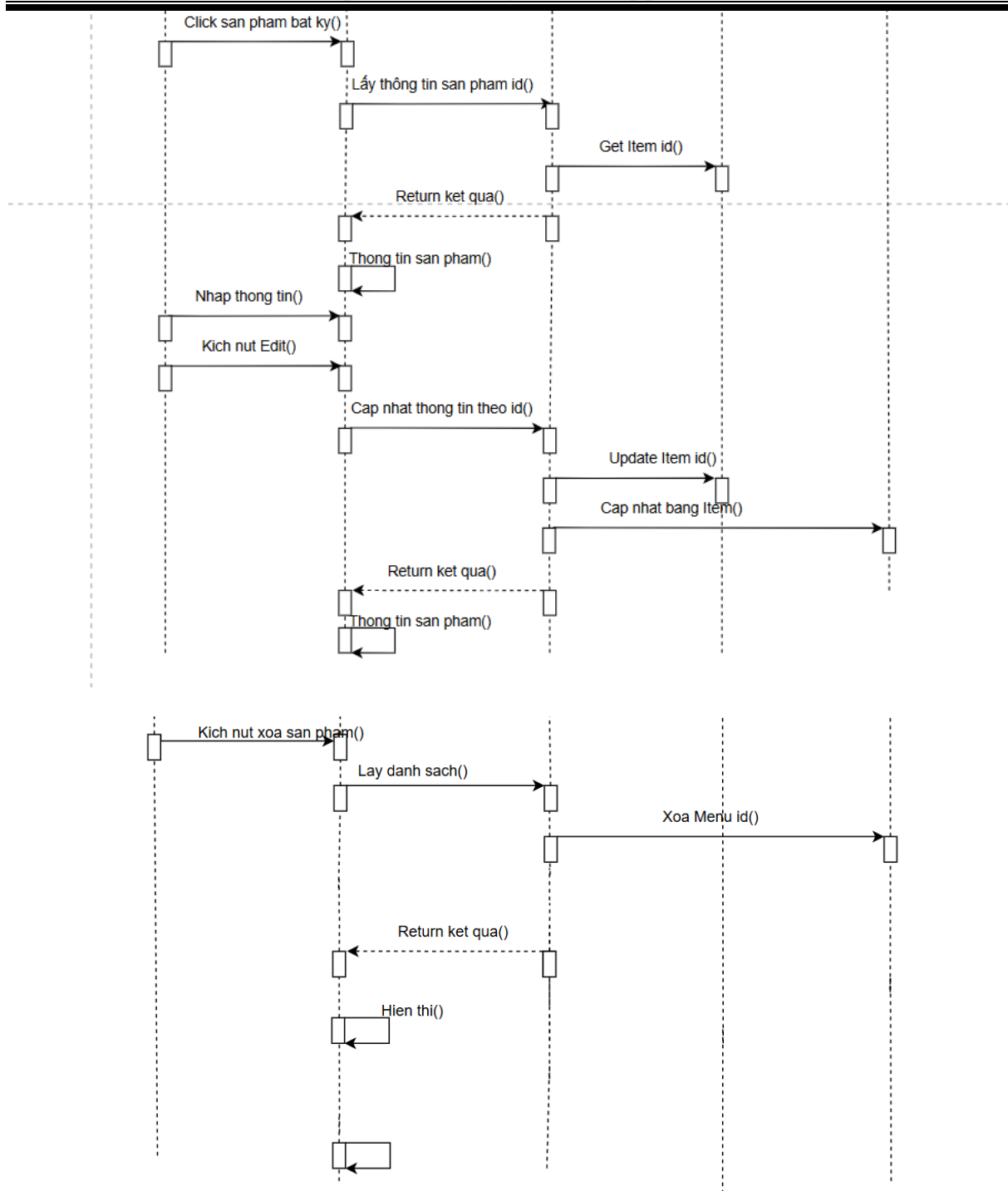
Hình 3-13: Biểu đồ trình tự chức năng quản lý sản phẩm
