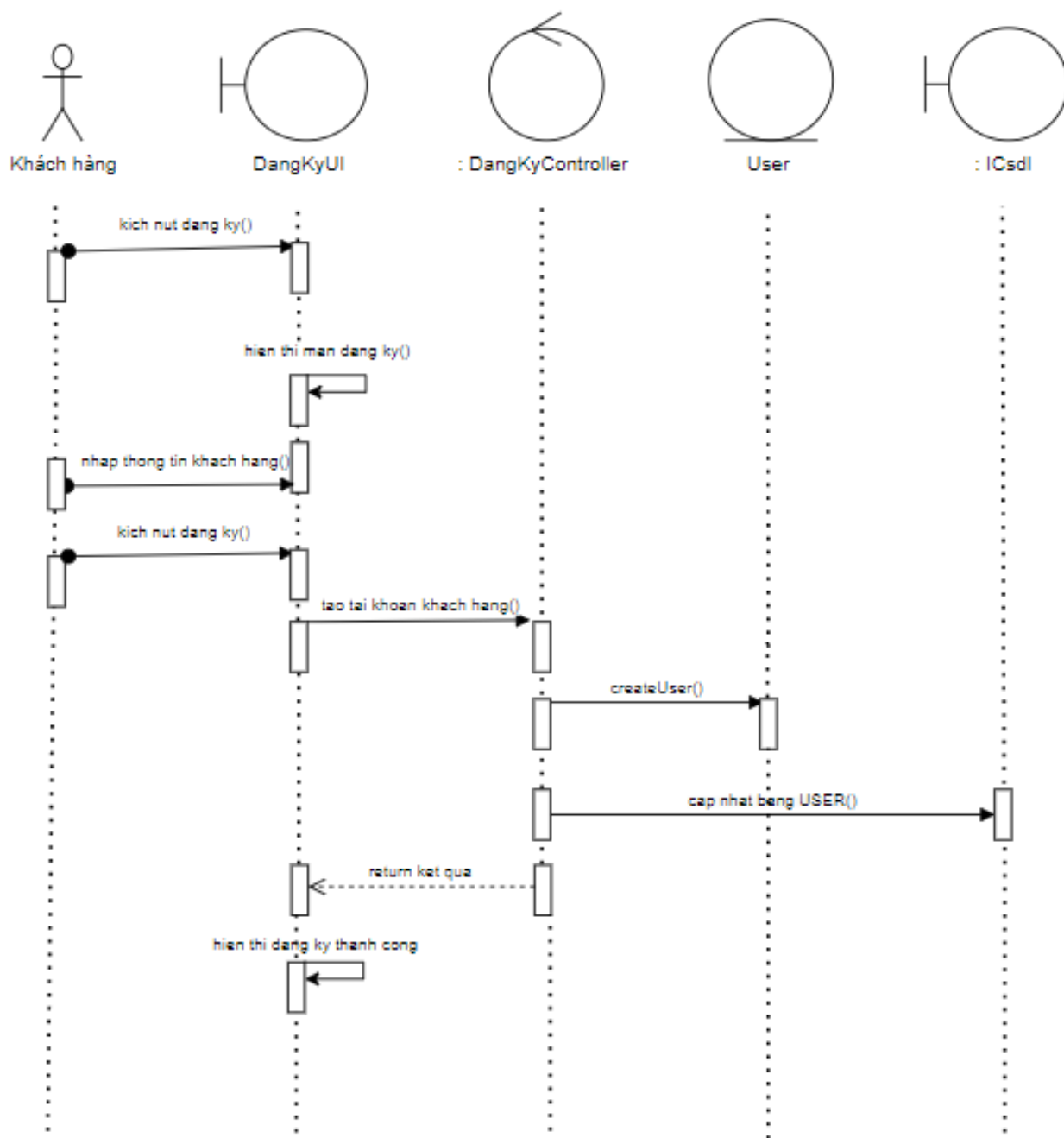
Hình 3-4: Biểu đồ trình tự chức năng đăng ký
