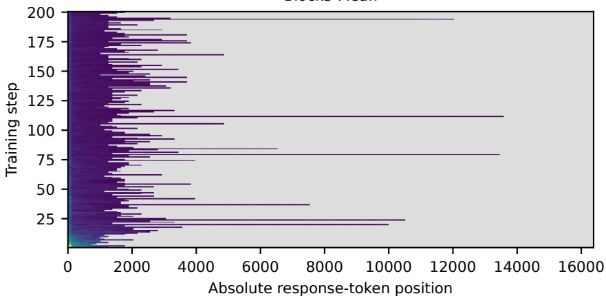
Token OPD
