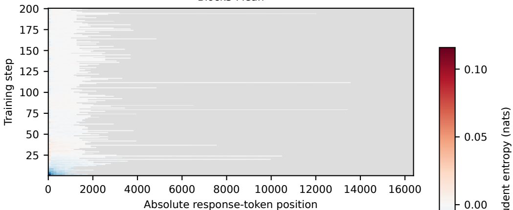
Token OPD
