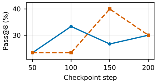
AIME25
