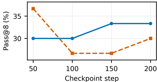
AMC23
