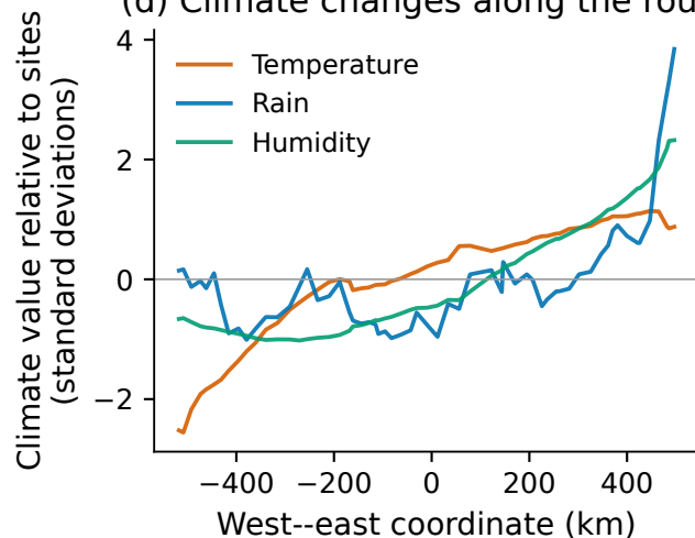
(d) Climate changes along the route
