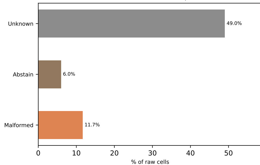
EXP-009: terminal failure mix (valid parse=0.883)
