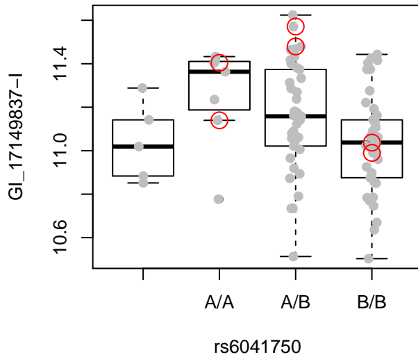
FKBP1A
