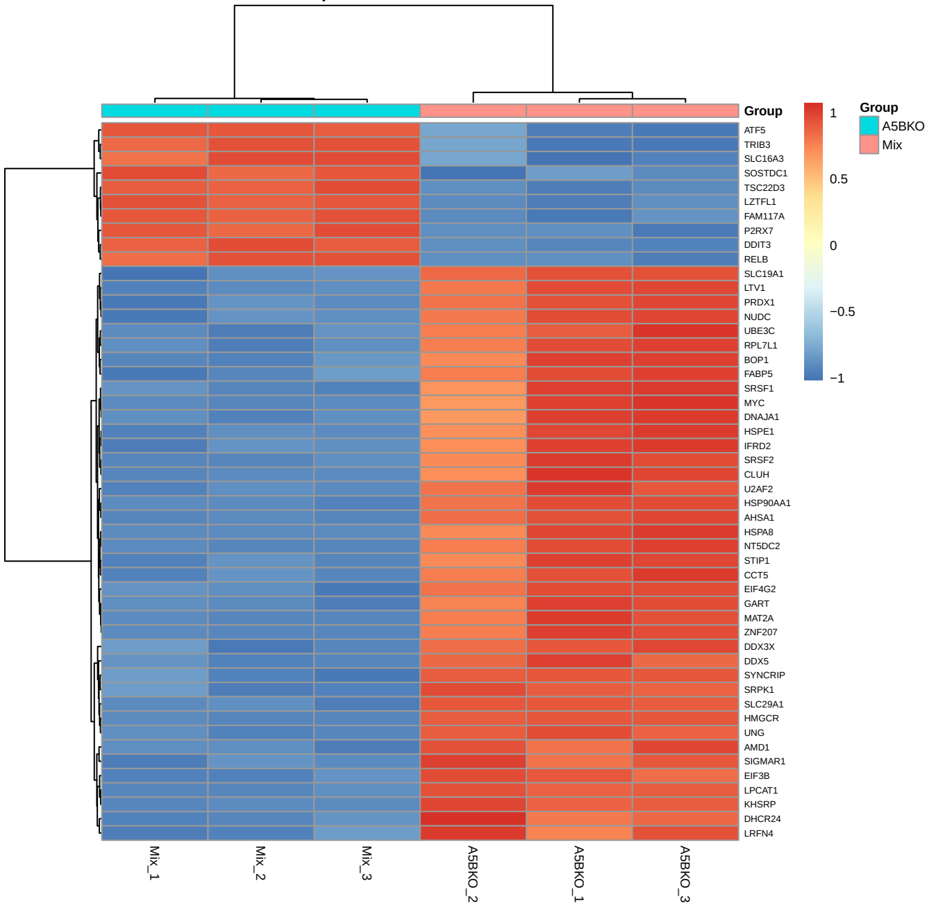
Top 50 DEGs: A5BKO_vs_Mix
