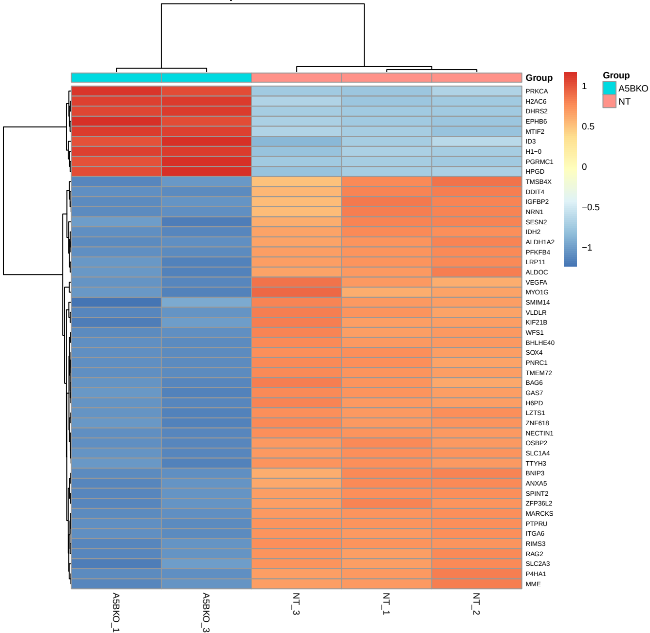
Top 50 DEGs: A5BKO_vs_NT
