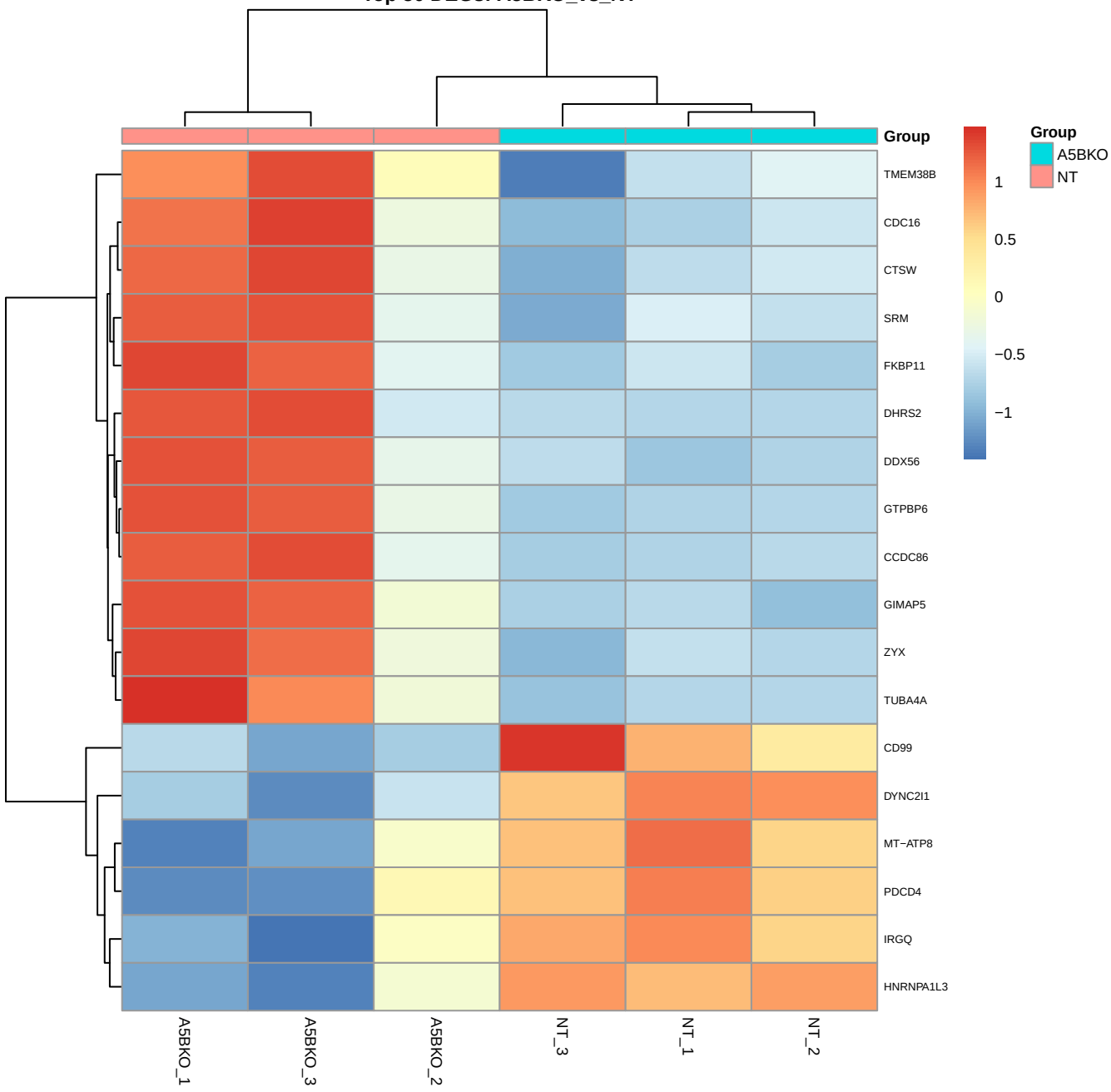
Top 50 DEGs: A5BKO_vs_NT
