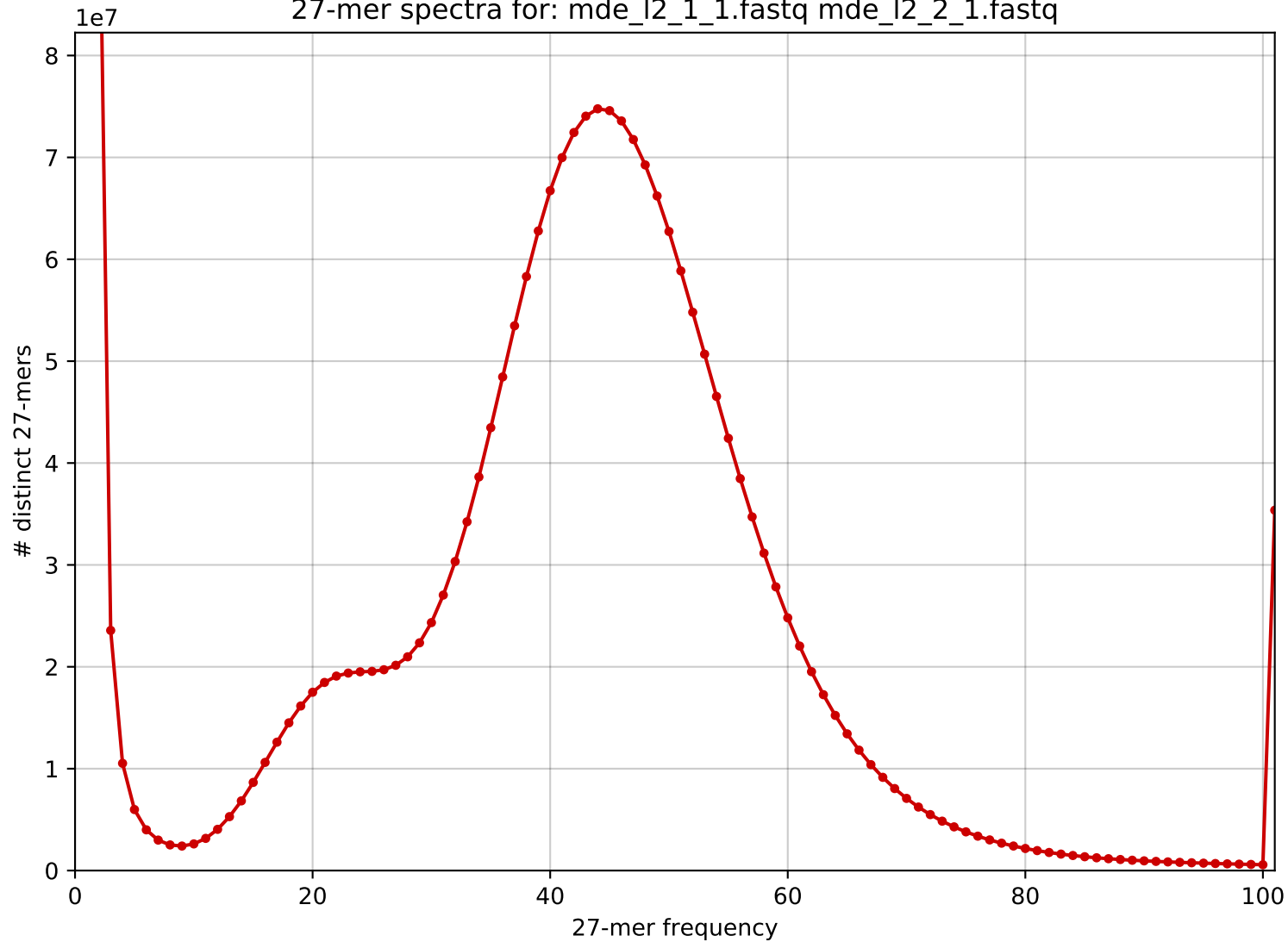
27-mer spectra for: mde_l2_1_1.fastq mde_l2_2_1.fastq
