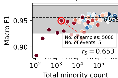
I LT1b | SOM classifier
