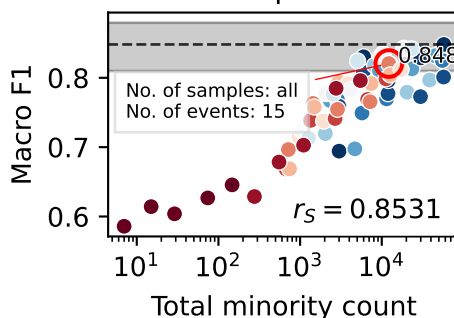
H LT1 | SOM classifier
