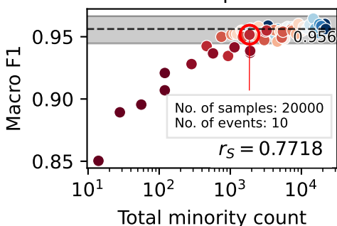
G Flowcyt | SOM classifier
