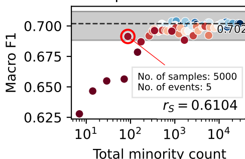
K LT2 | SOM classifier
