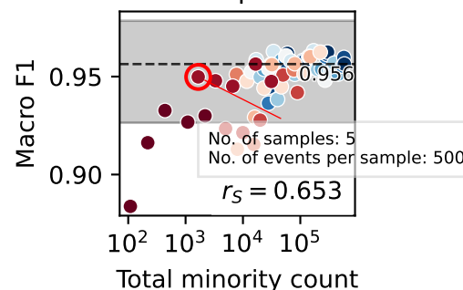
I LT1b | SOM classifier
