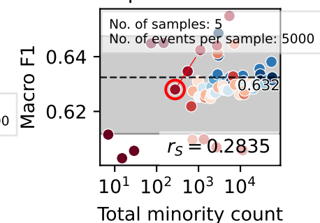
K LT2 | SOM classifier
