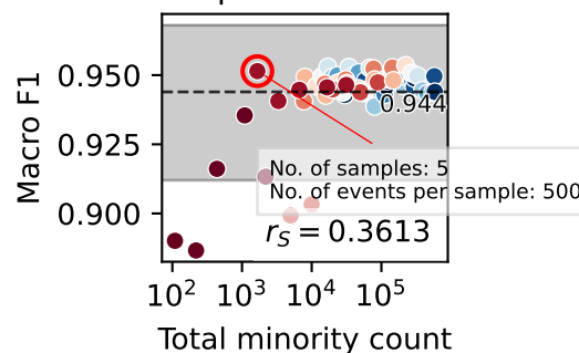
L LT2b | SOM classifier
