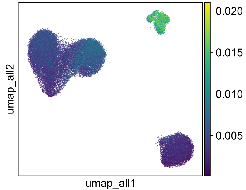
naive_all
