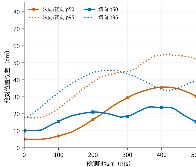
A 原地旋转 8 rad/s
