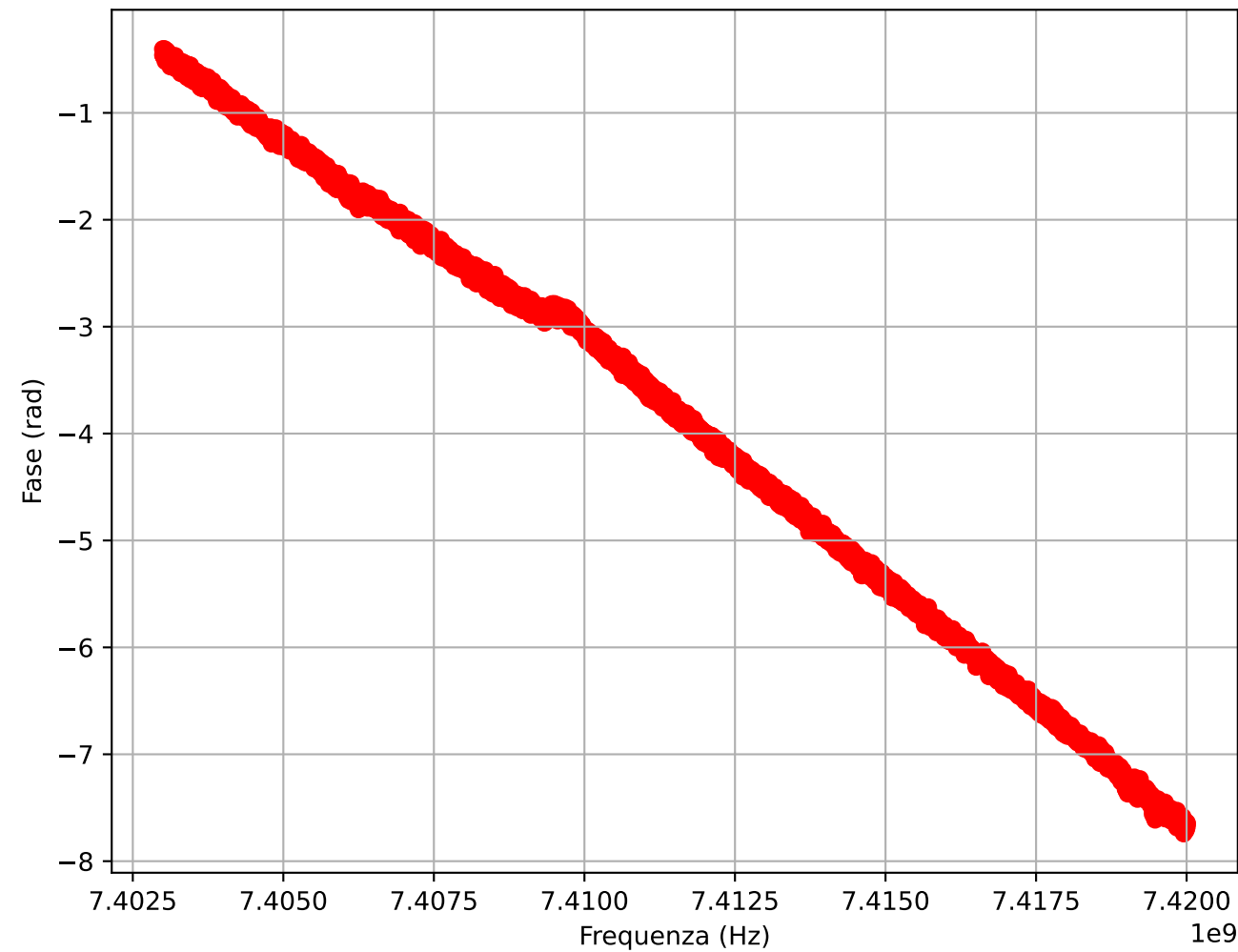
Fase S21
