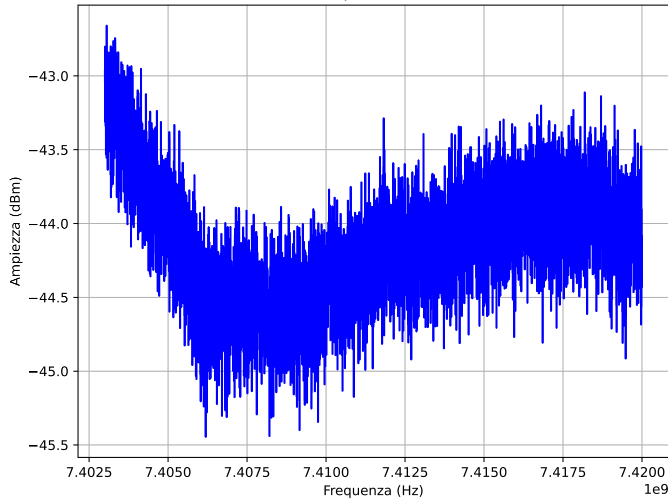
Ampiezza S21
