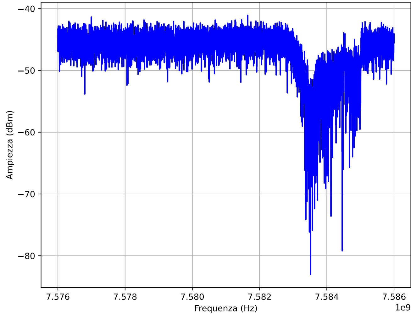
Ampiezza S21
