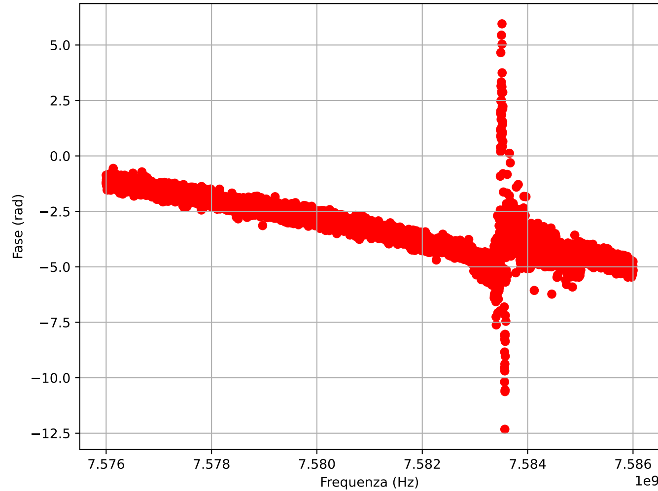
Fase S21
