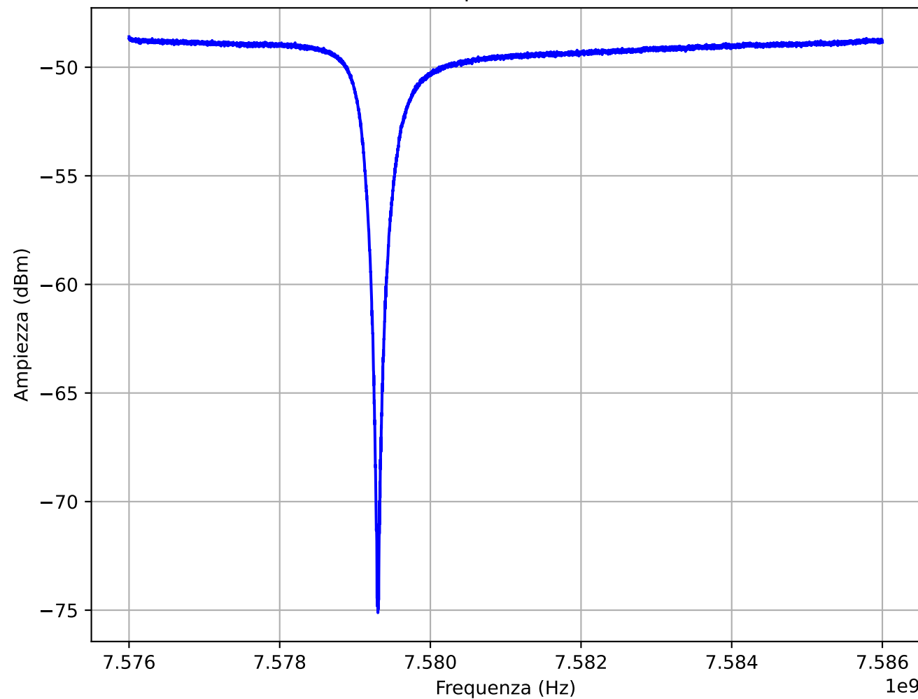
Ampiezza S21
