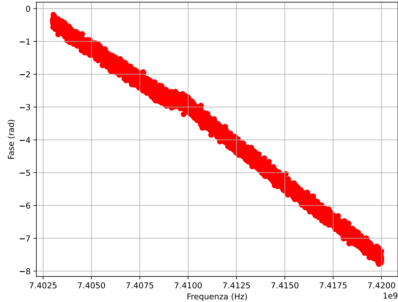
Fase S21
