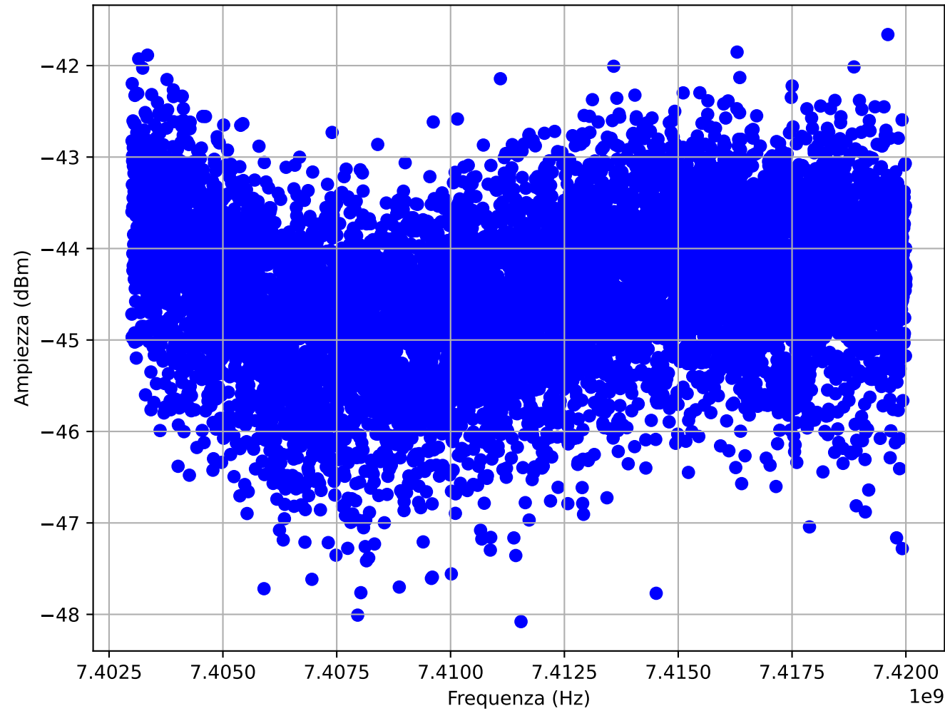
Ampiezza S21
