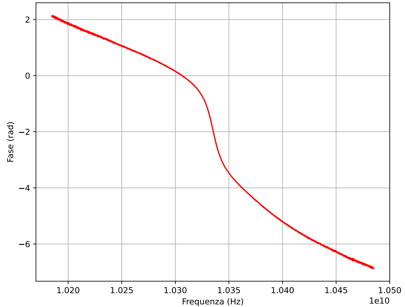
Fase S21
