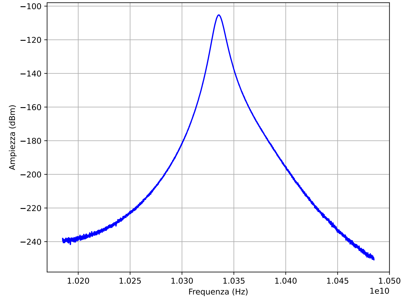
Ampiezza S21
