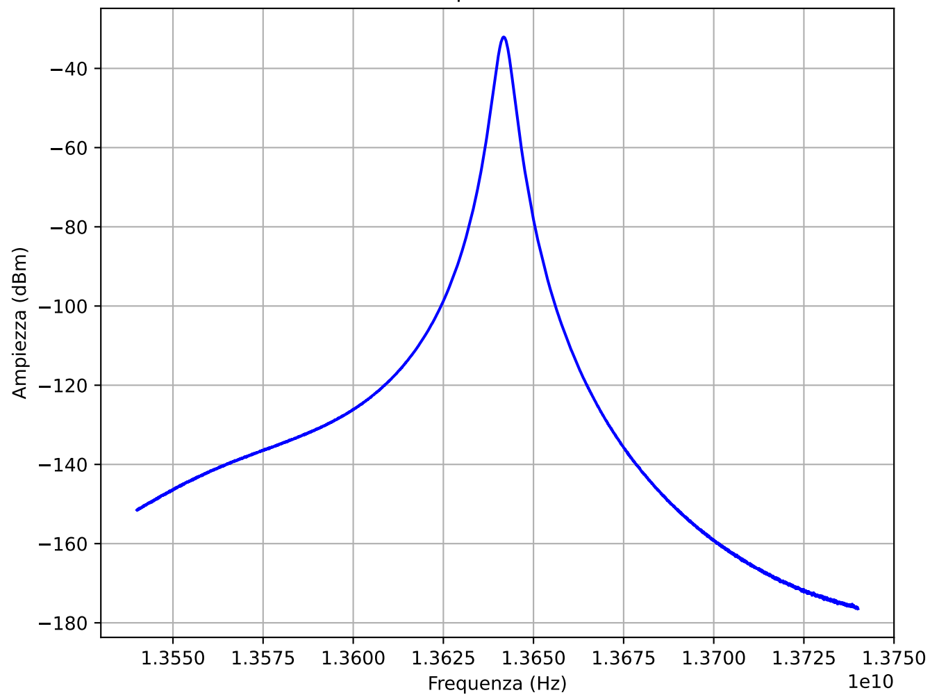
Ampiezza S21
