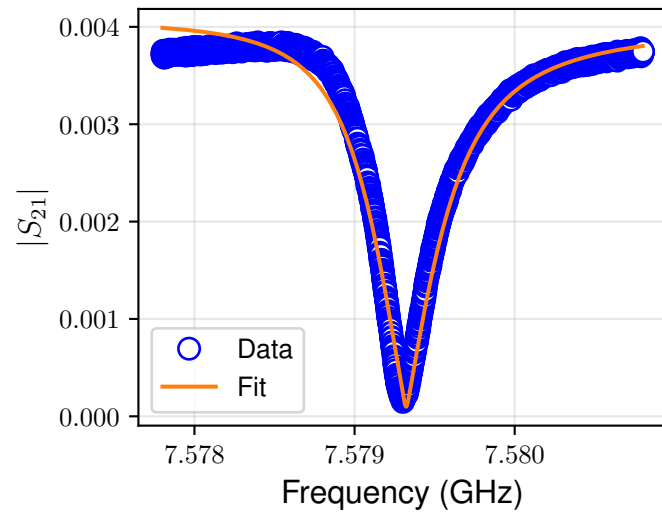
Magnitude
