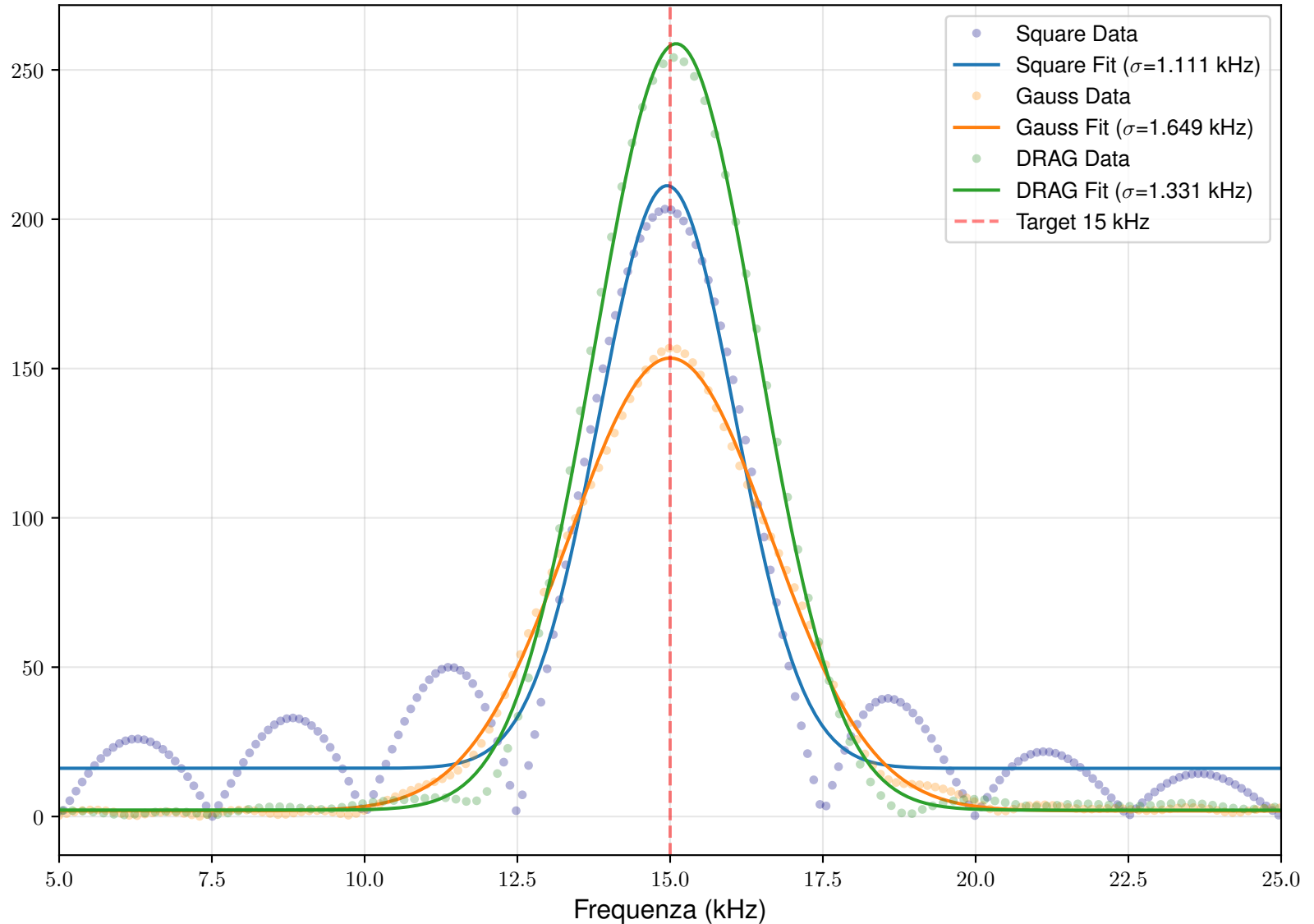
Confronto Fit Gaussiani su Spettri
