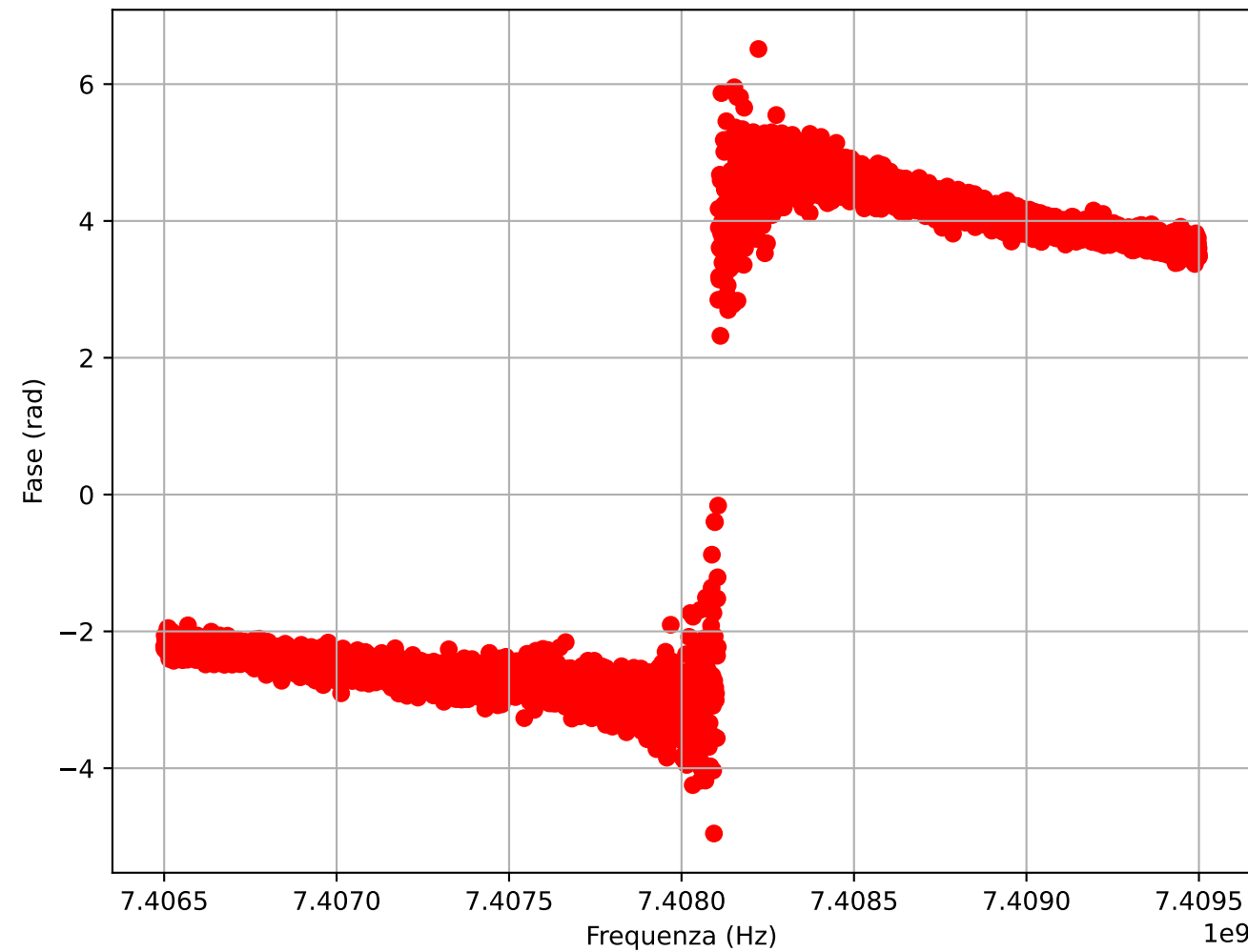
Fase S21
