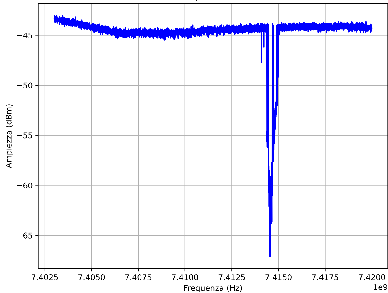
Ampiezza S21
