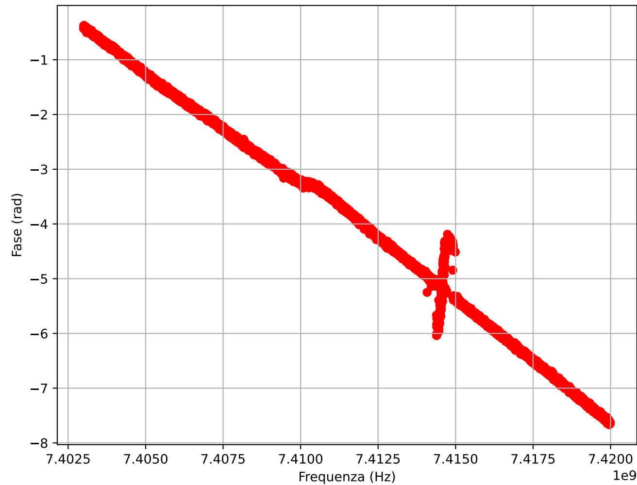
Fase S21
