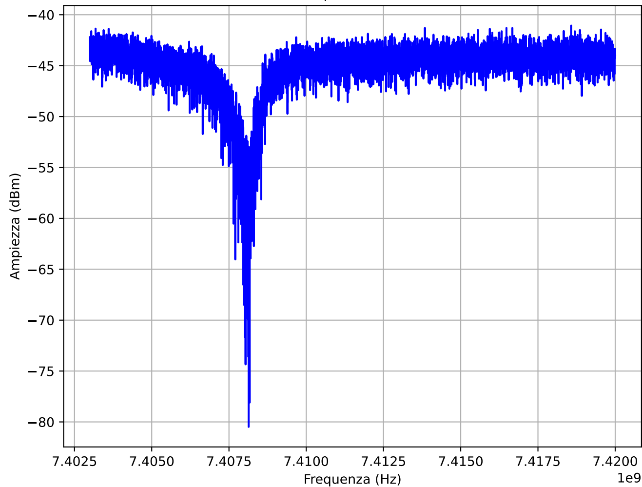
Ampiezza S21
