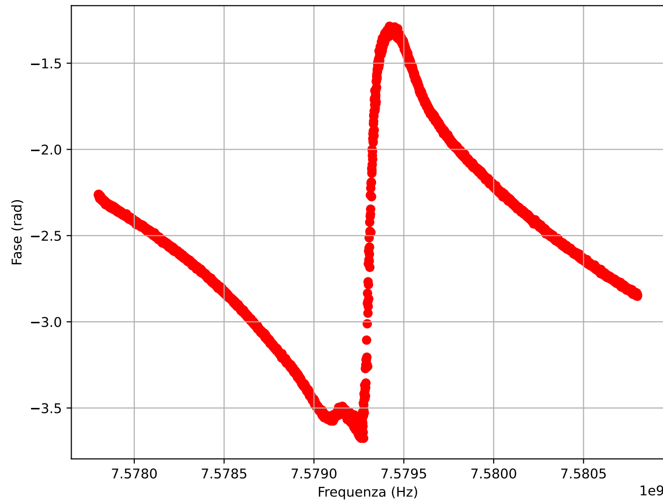
Fase S21
