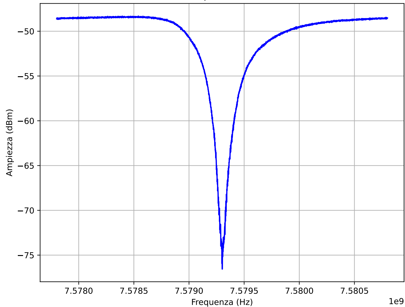
Ampiezza S21
