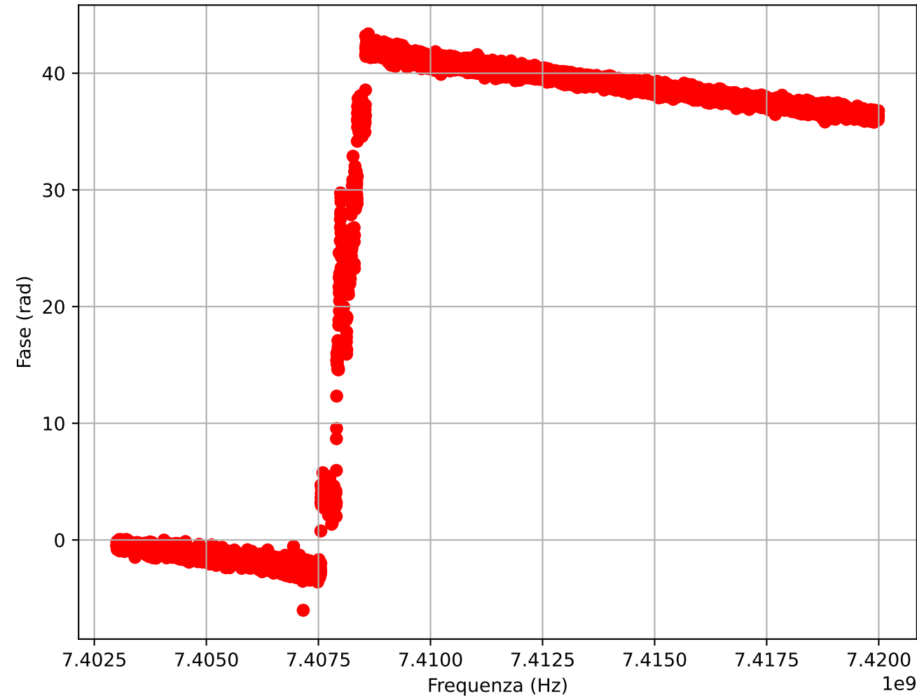
Fase S21
