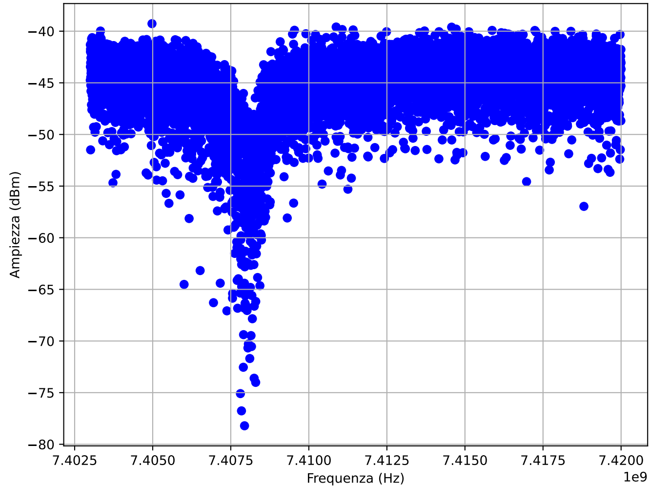
Ampiezza S21
