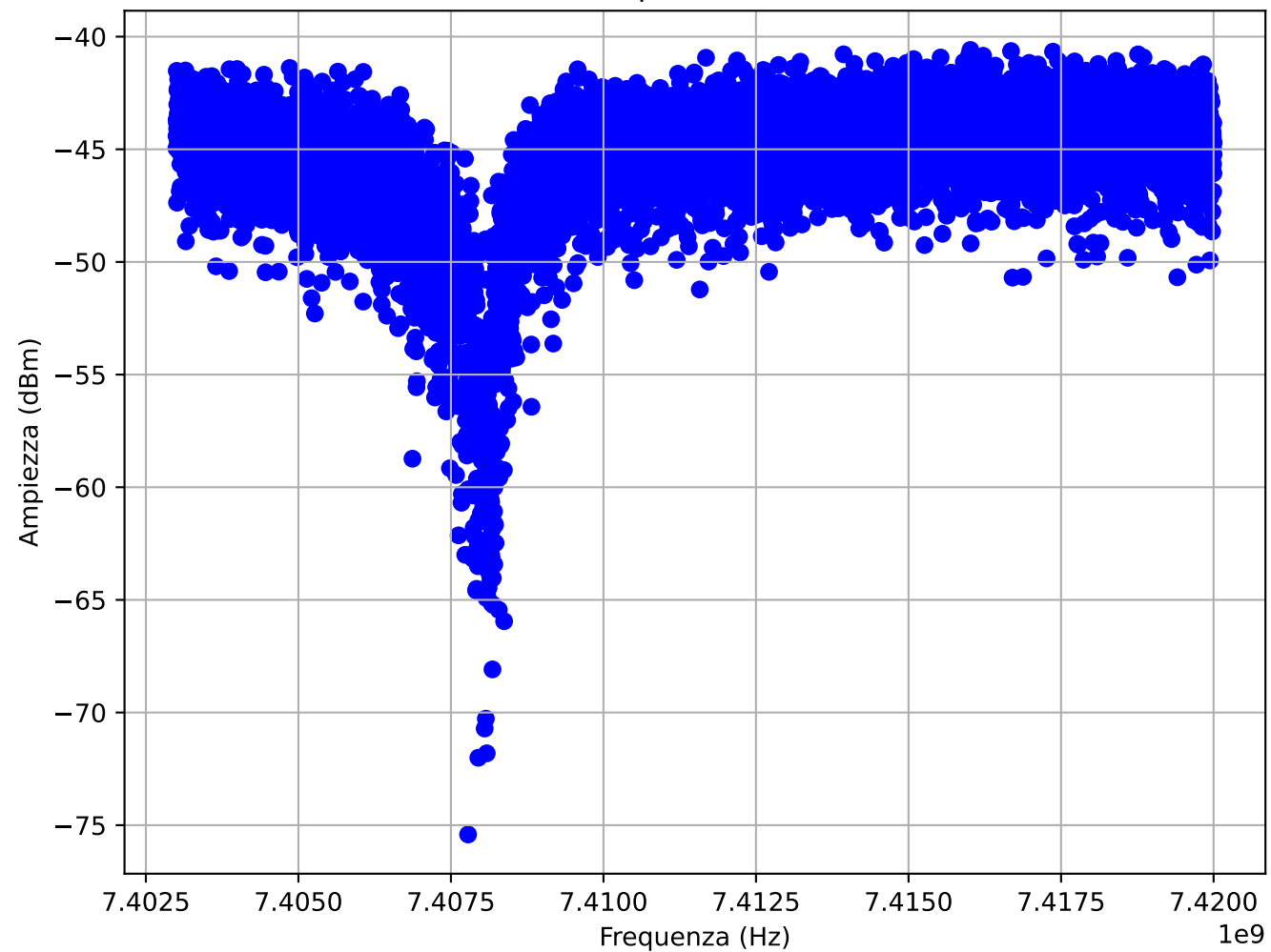
Ampiezza S21
