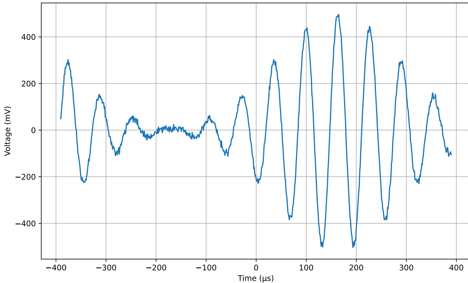
PICO DRAG Pulse - Carrier: 15.0 kHz
