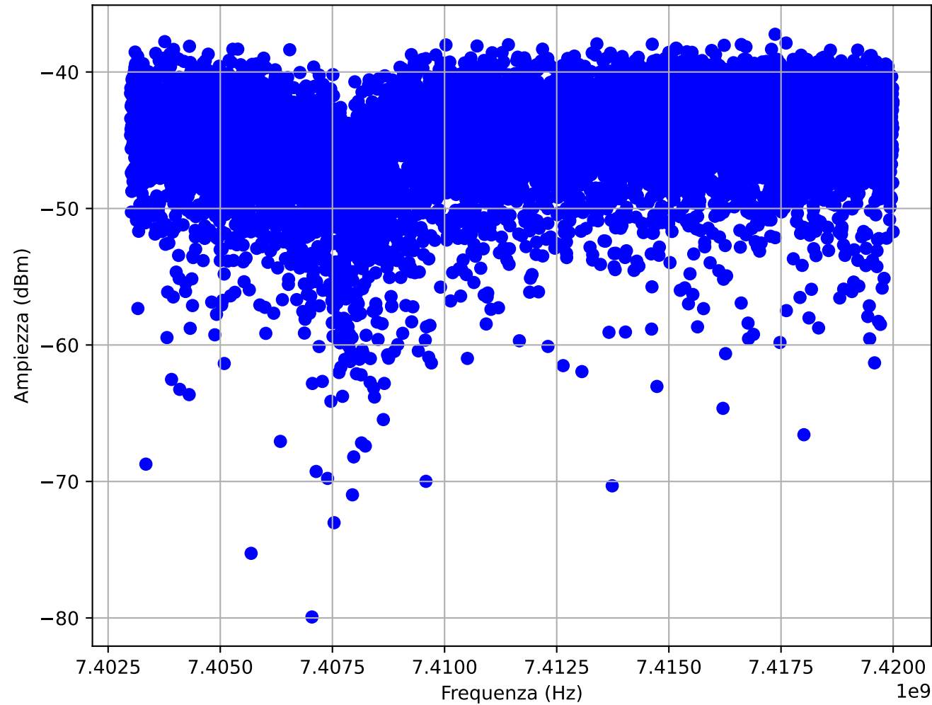
Ampiezza S21
