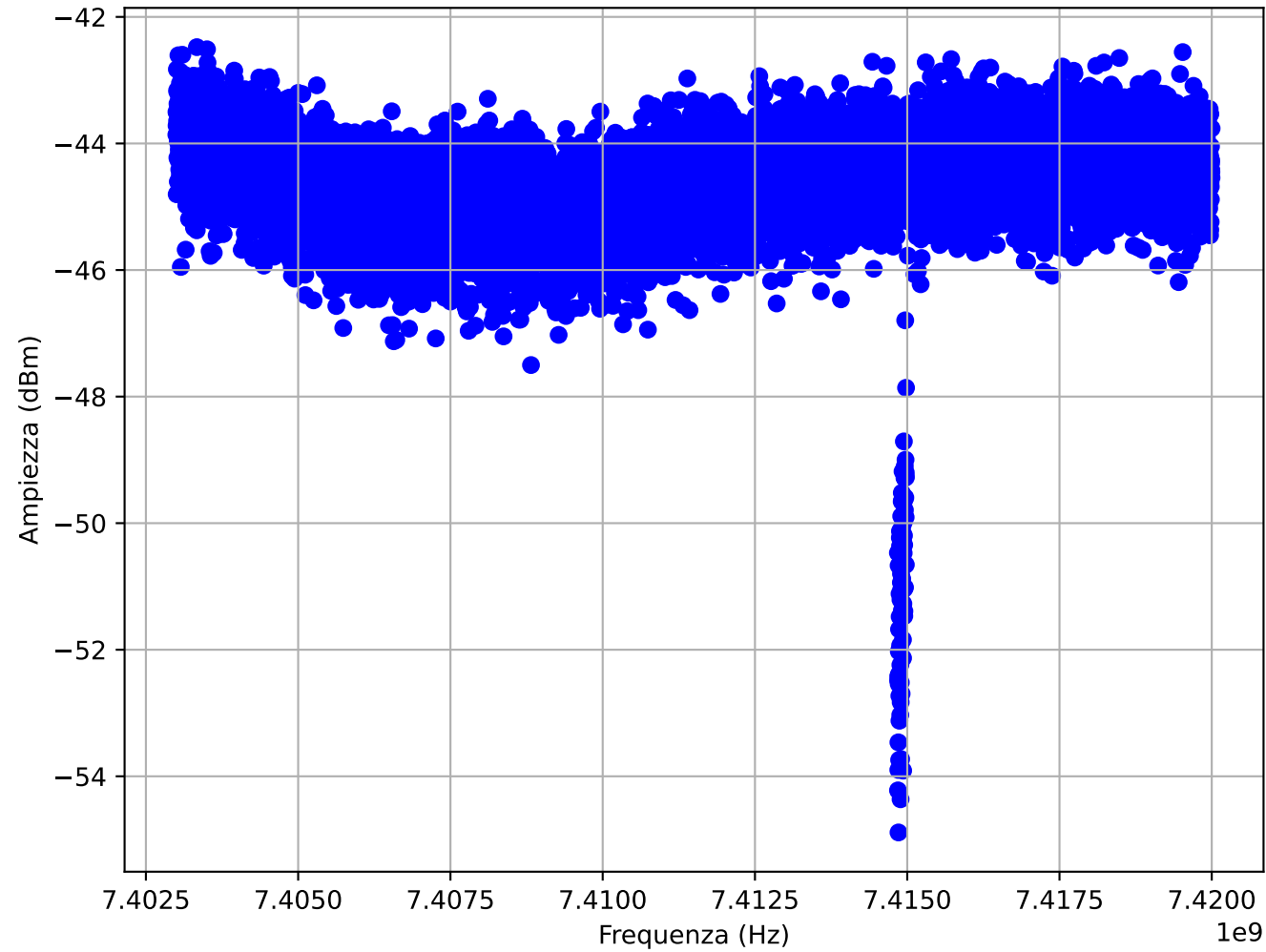
Ampiezza S21
