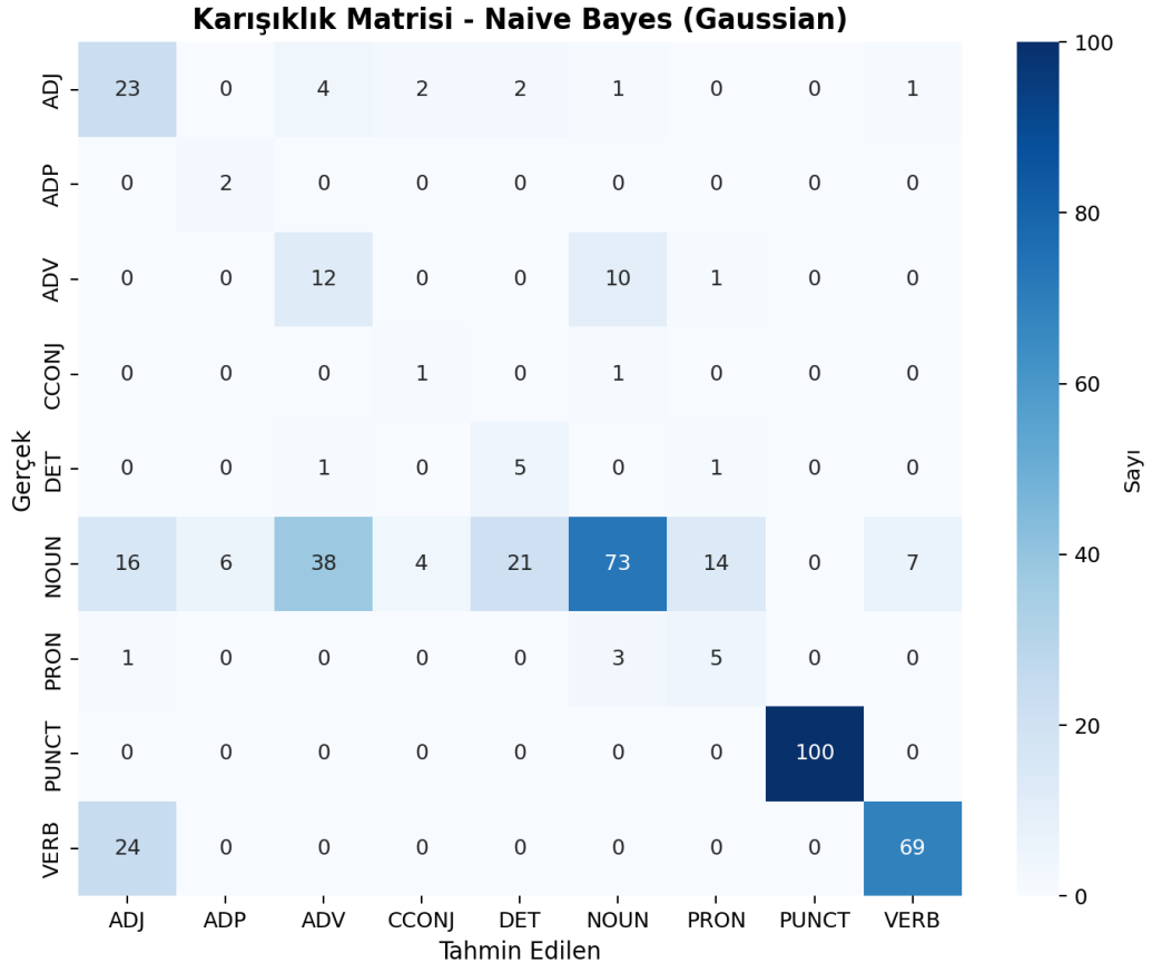
Şekil 5: Naive Bayes — Karışıklık Matrisi
