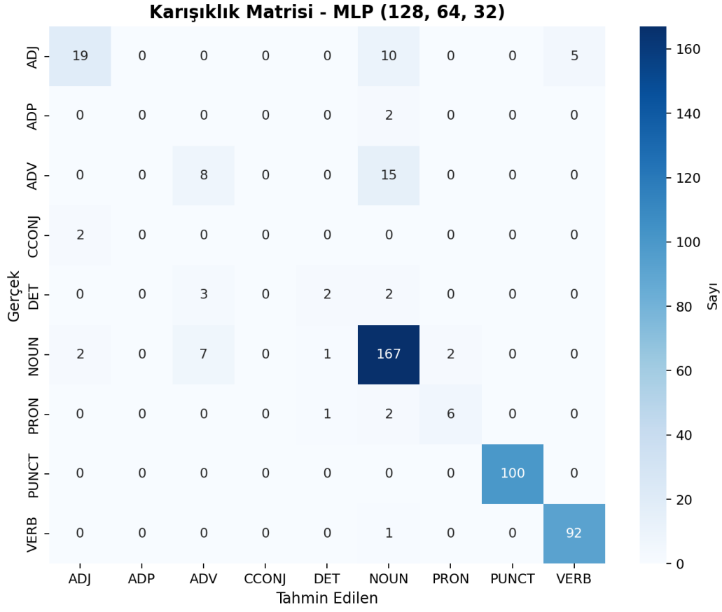
Şekil 4: MLP — Karışıklık Matrisi
