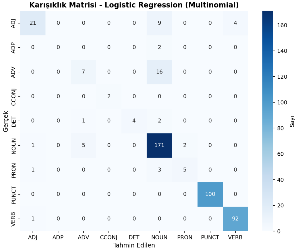
Şekil 3: Logistic Regression — Karışıklık Matrisi
