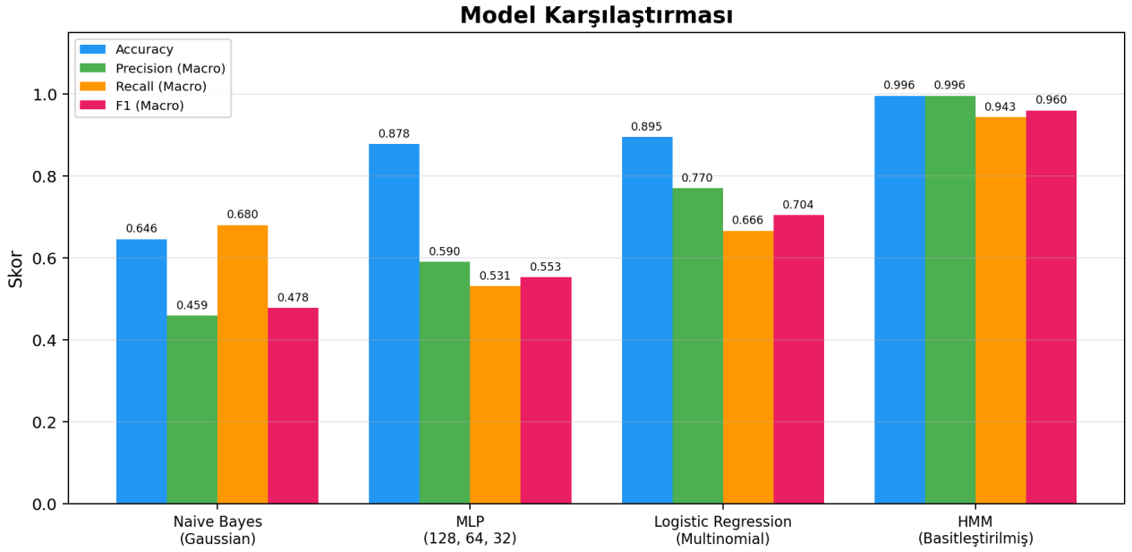
Şekil 1: Model karşılaştırma grafiği (Accuracy, Precision, Recall, F1)
