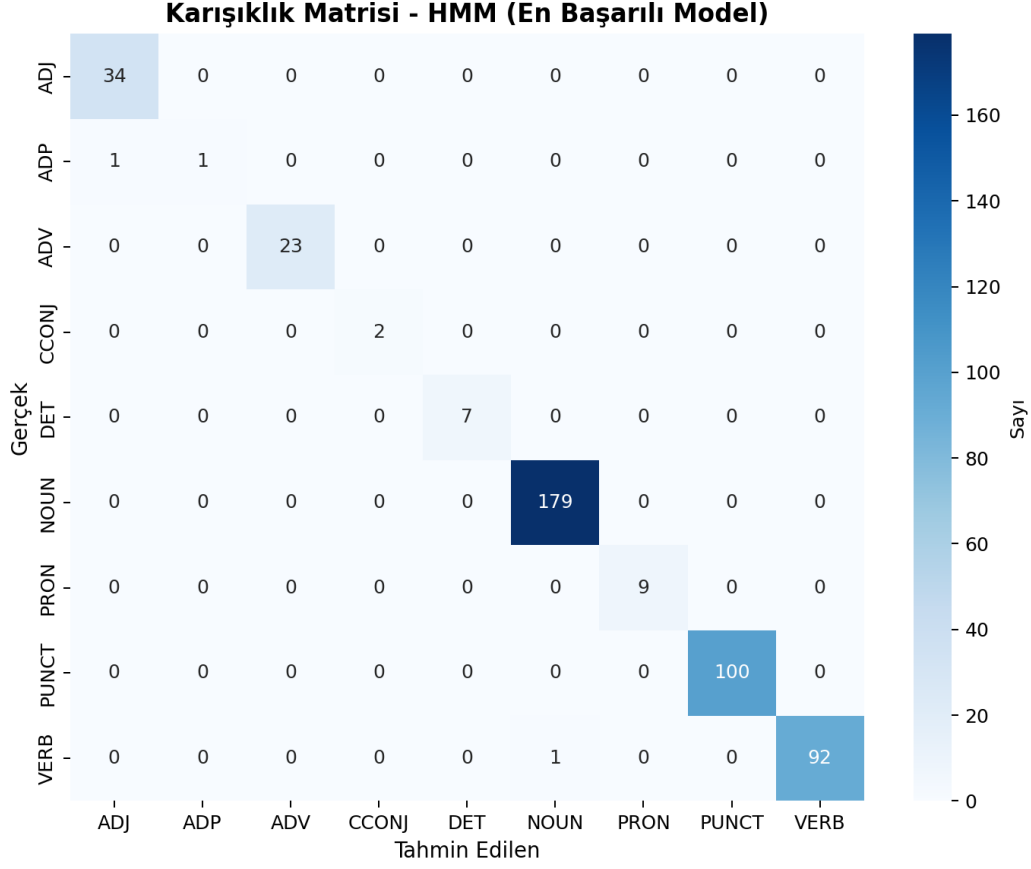
Şekil 2: HMM — Karışıklık Matrisi (En Başarılı Model)
