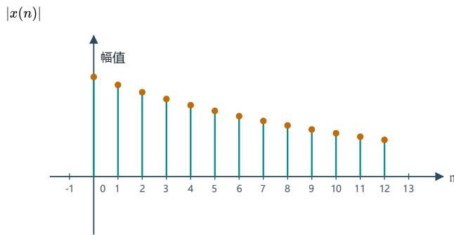
复指数序列的模
