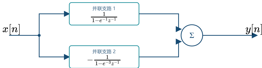
脉冲响应不变法得到的 IIR 并联型结构
