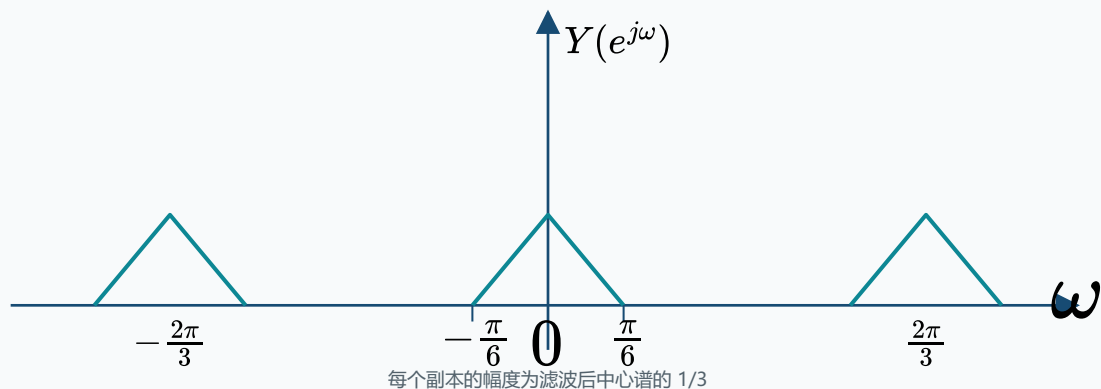
周期采样后的频谱复制
