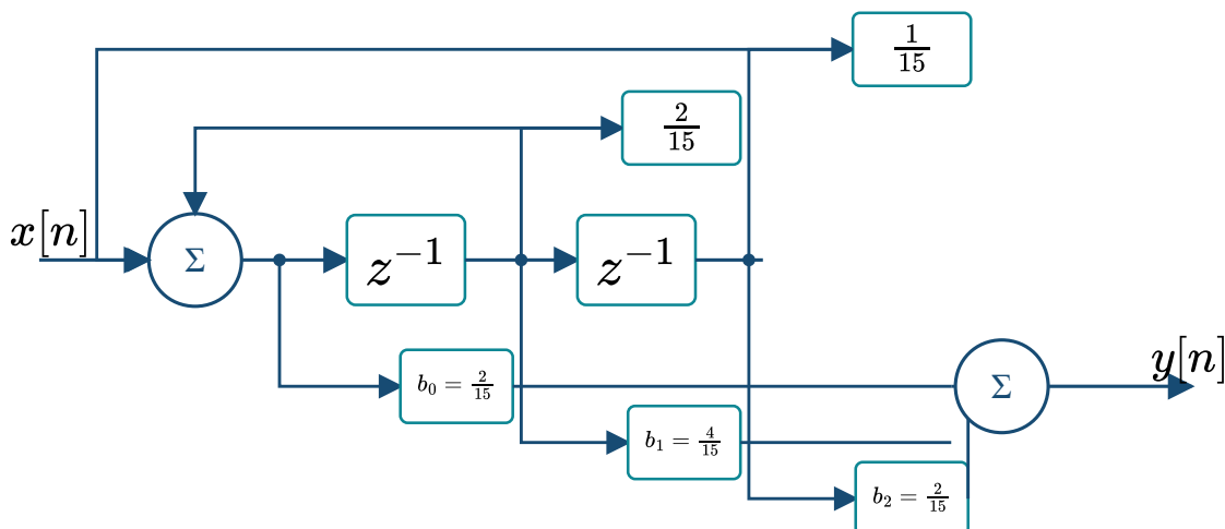
双线性变换得到的 IIR 直接 II 型结构
