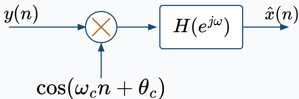
(c) 相干解调与低通恢复
