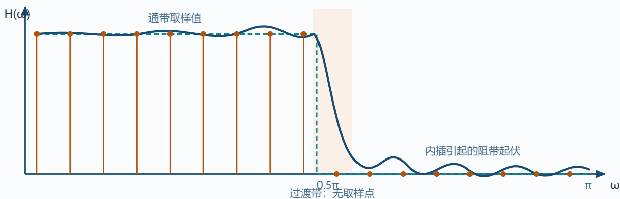
频率采样点与过渡带起伏
