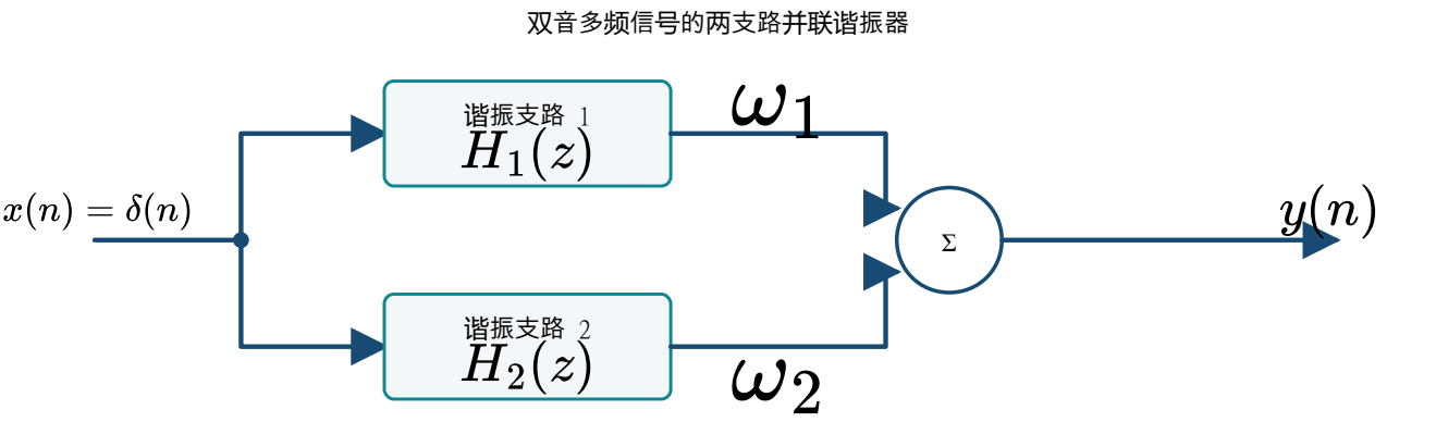
图 5-3 并联型结构示例：双音多频信号
