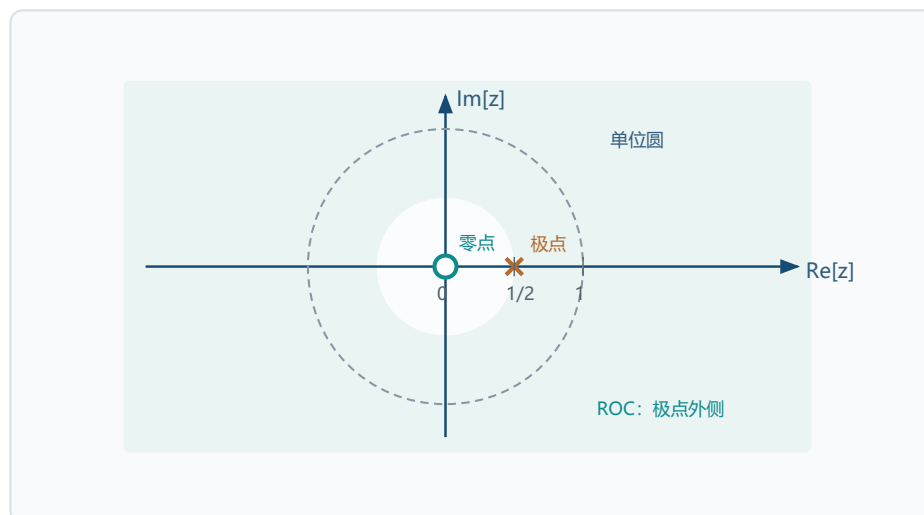
零点、极点、单位圆与因果收敛域。
