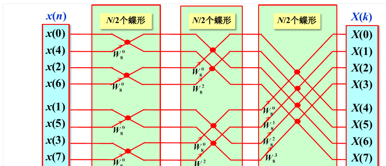
8 点 DFT 按时间抽取的 2-FFT 分解流程图
