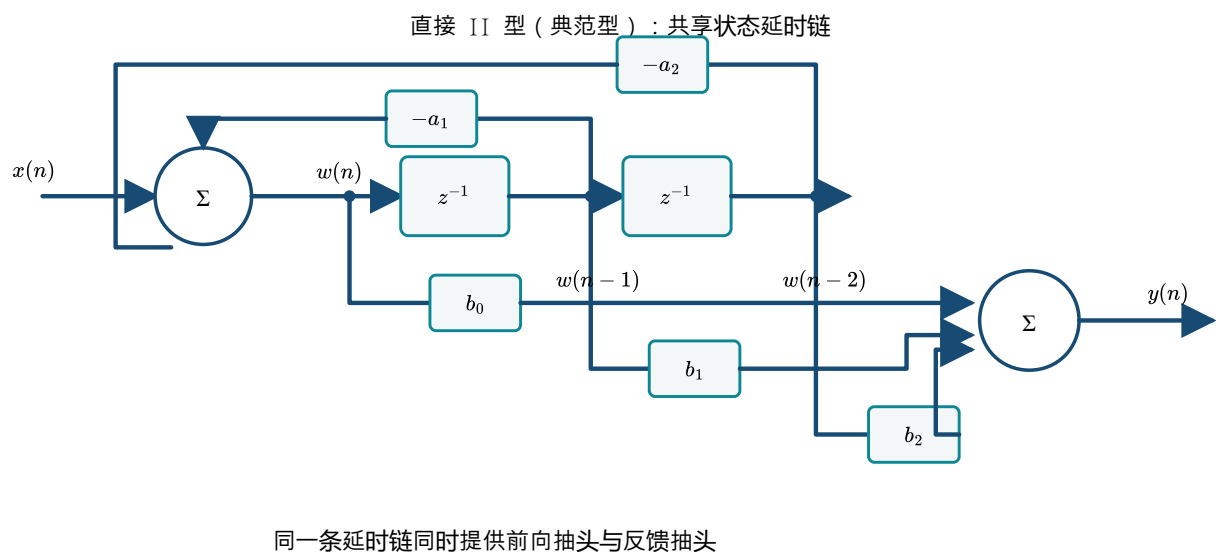
图 5-2 IIR 直接 II 型（典型型）结构
