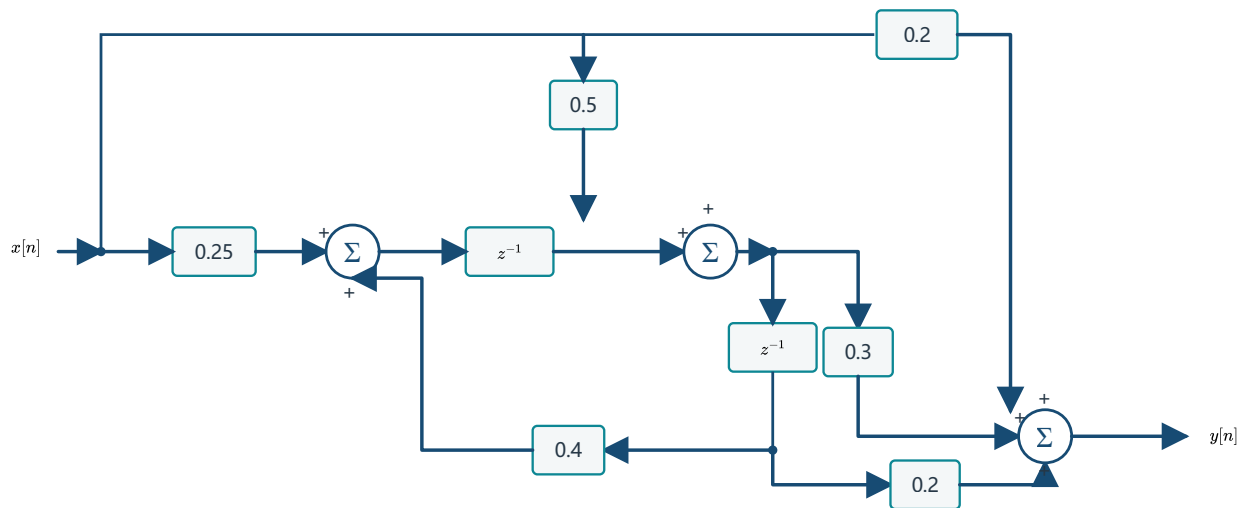
离散系统结构图
