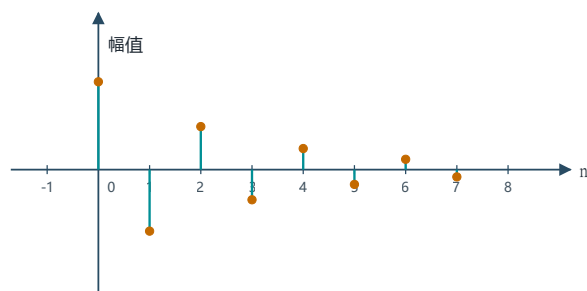
正负交替的实指数序列
